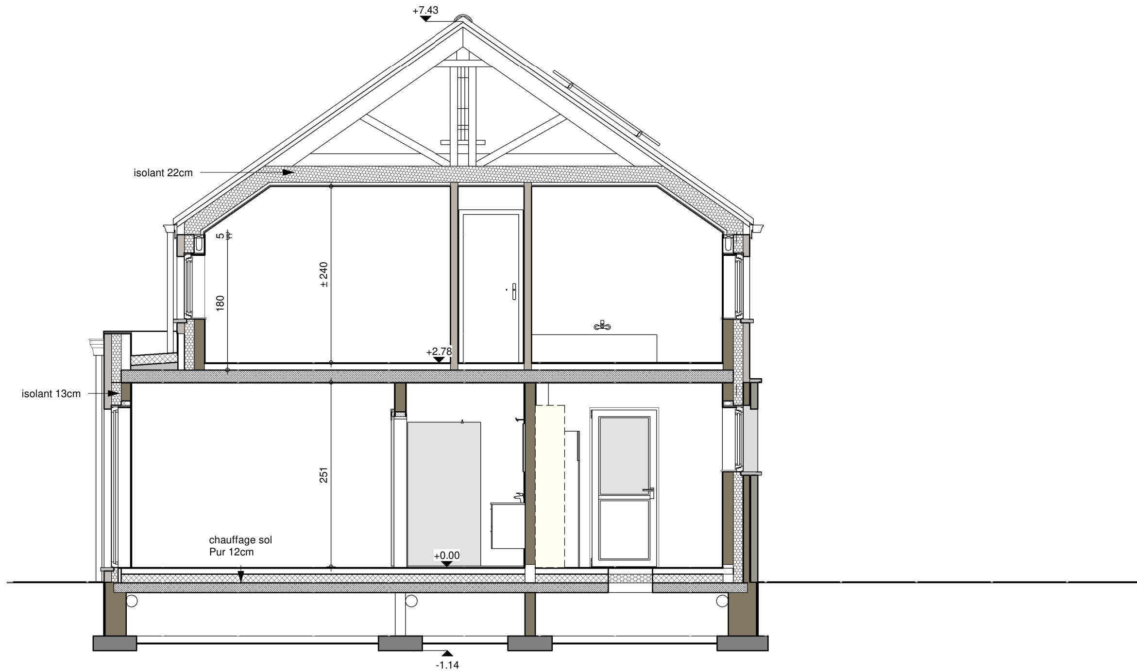
COUPE AA
