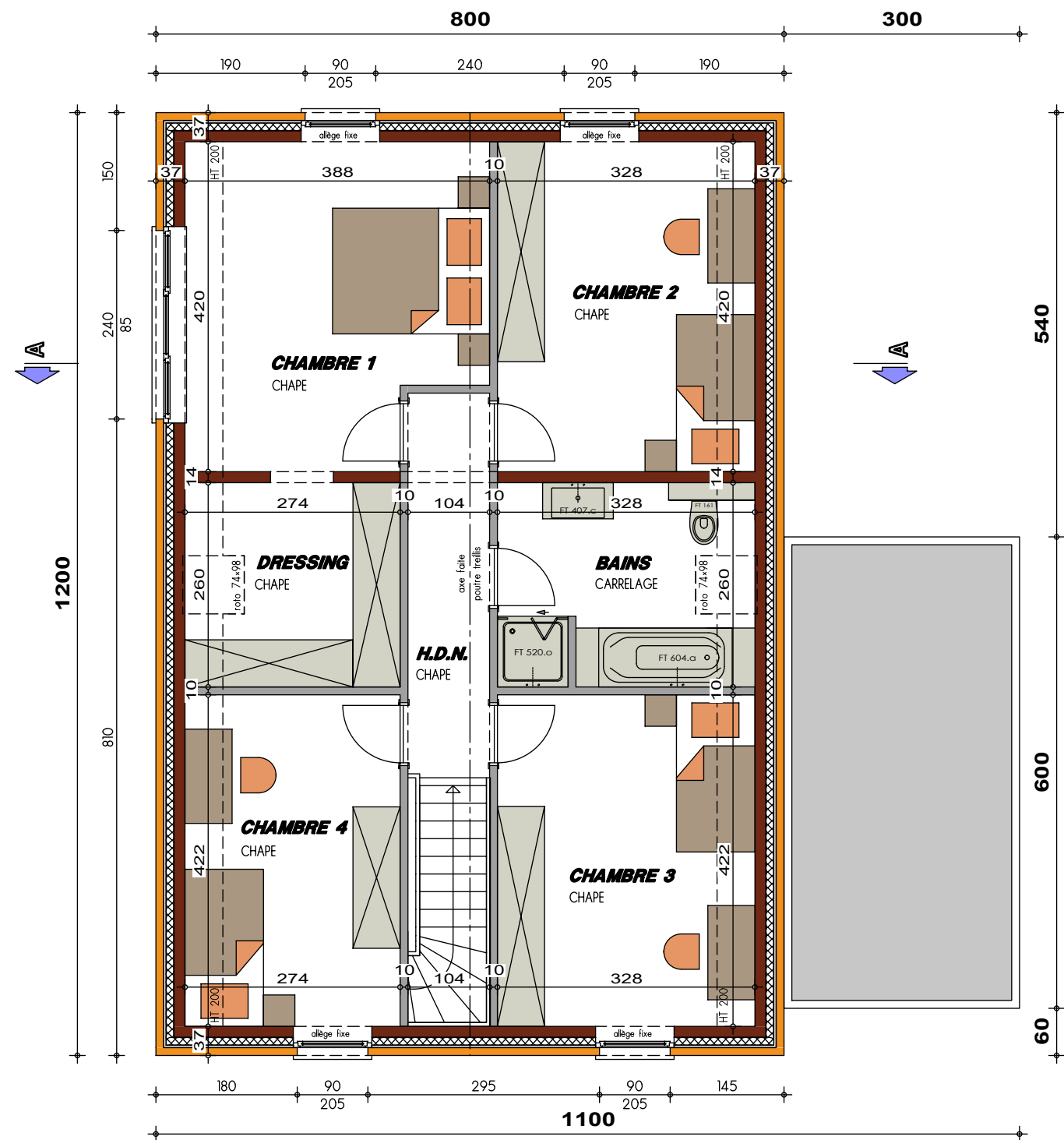
PLAN ETAGE
