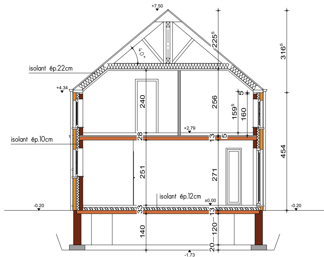
COUPE AA
