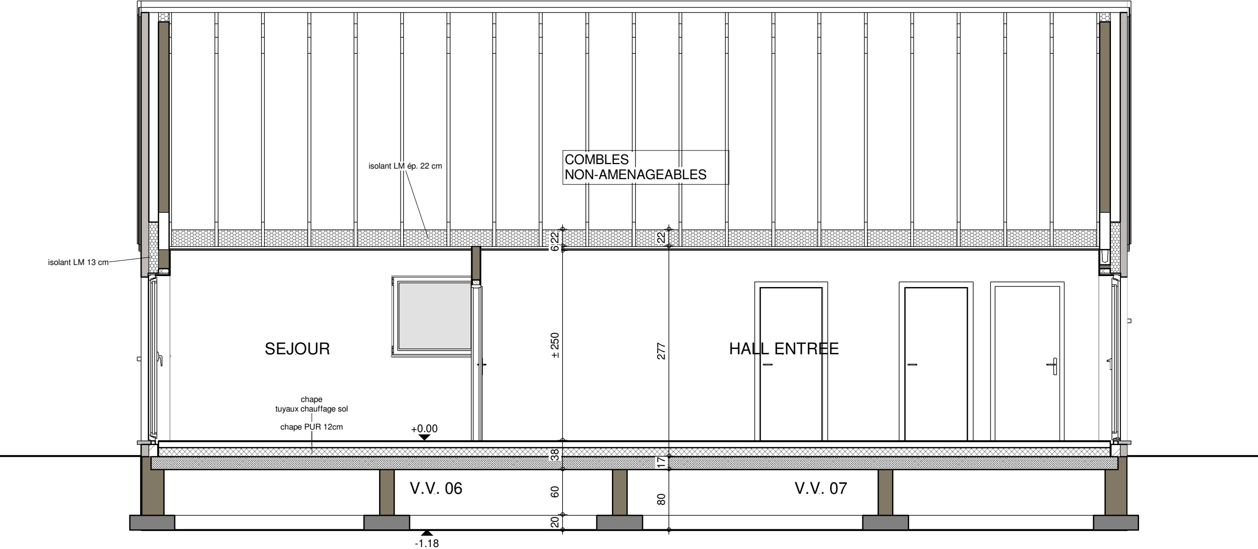
COUPE AA
