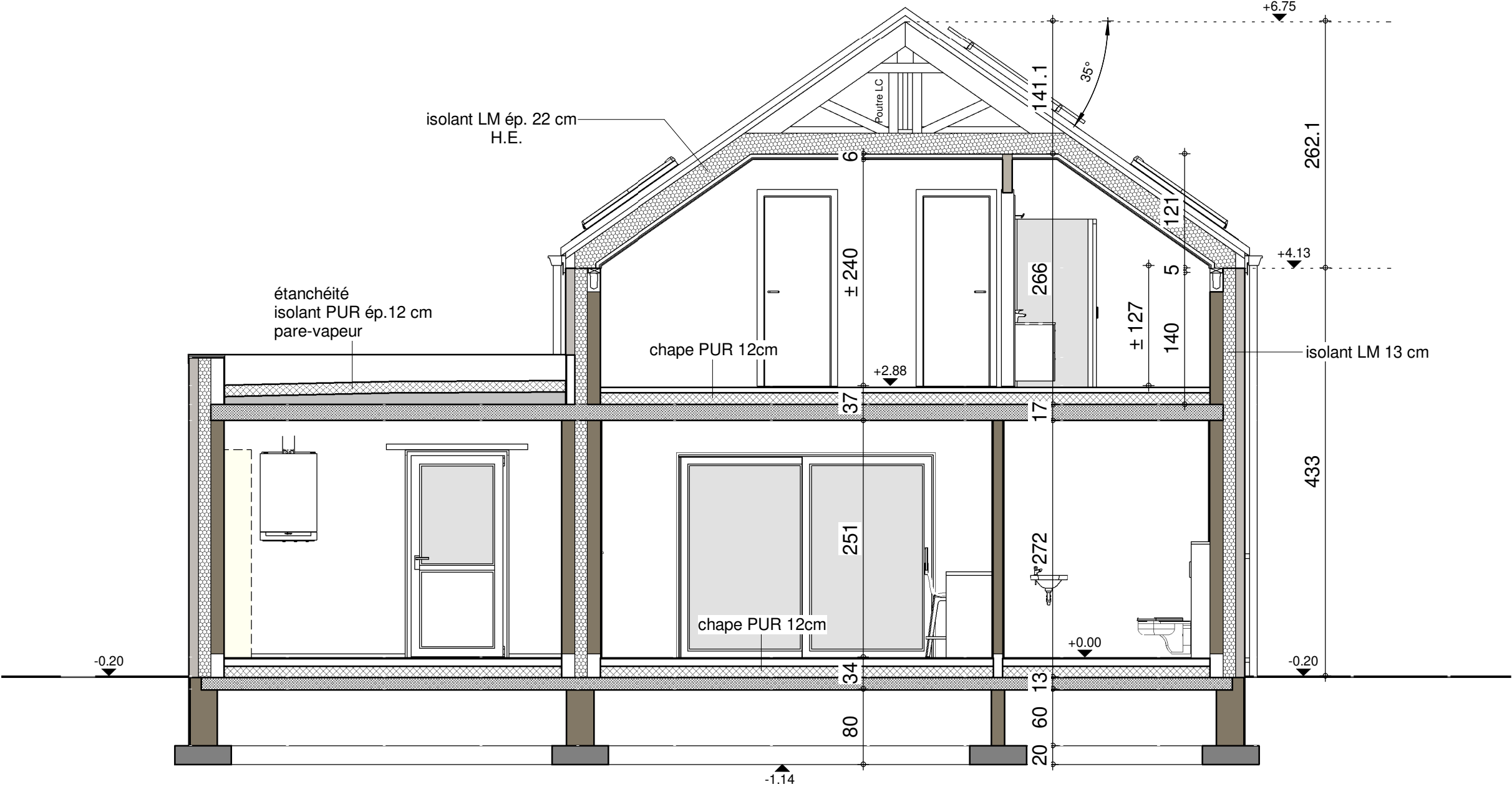
COUPE AA
