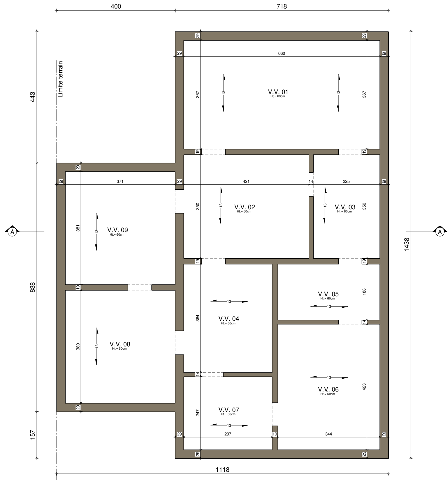
SOUS-SOL
