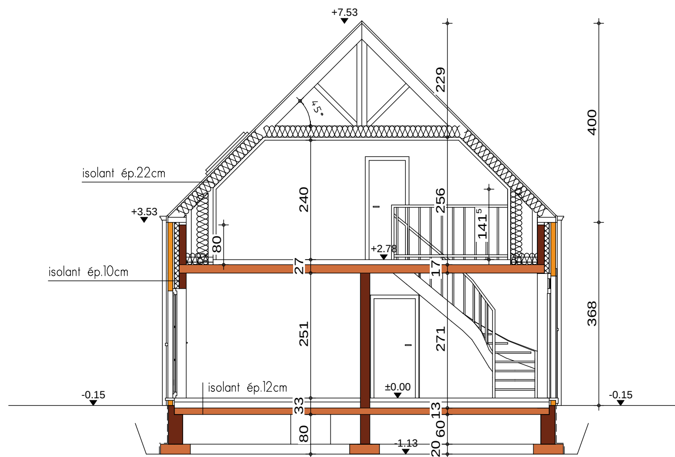
COUPE AA
