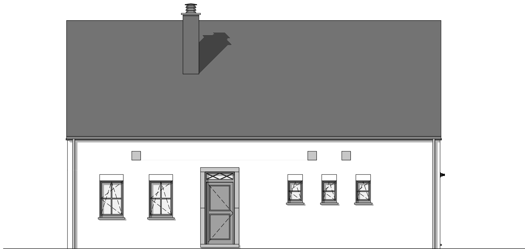
FACADE AVANT
