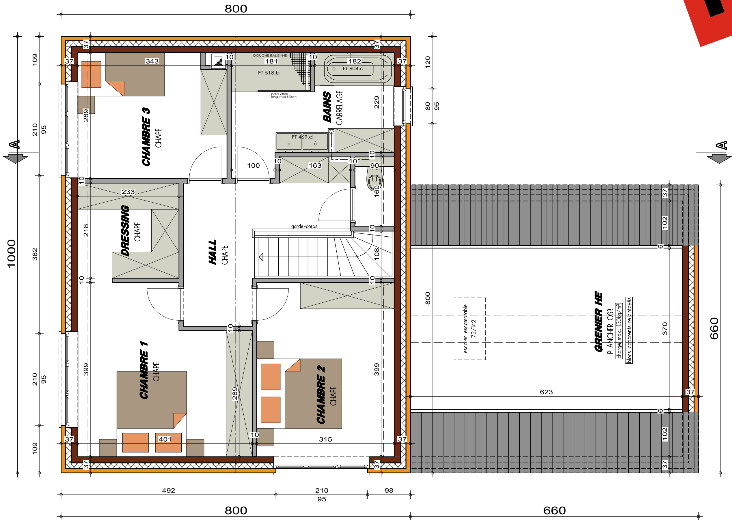
PLAN ETAGE
