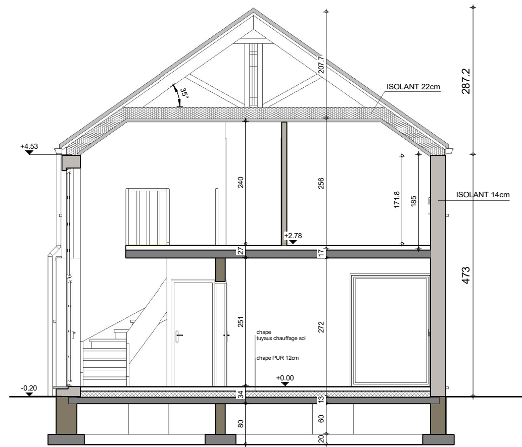
COUPE AA
