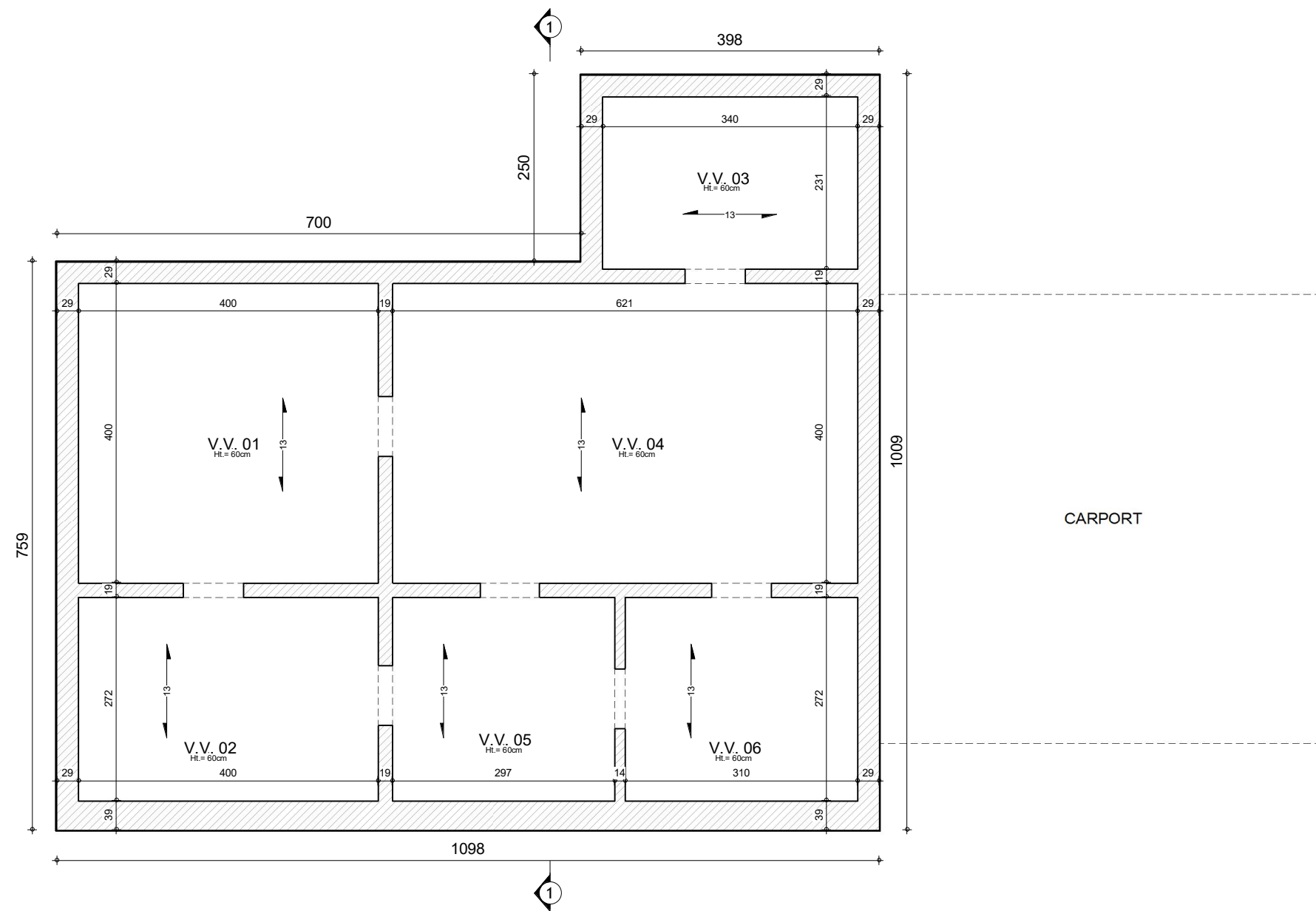
SOUS-SOL : Egouttage
