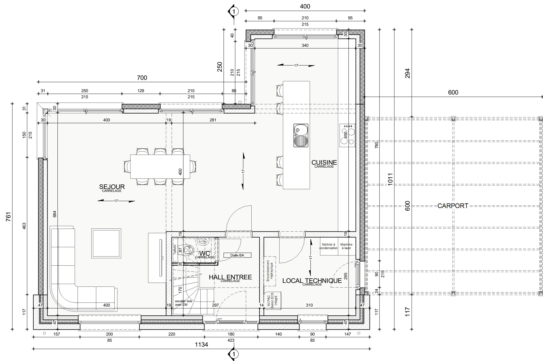
REZ-DE-CHAUSSEE
