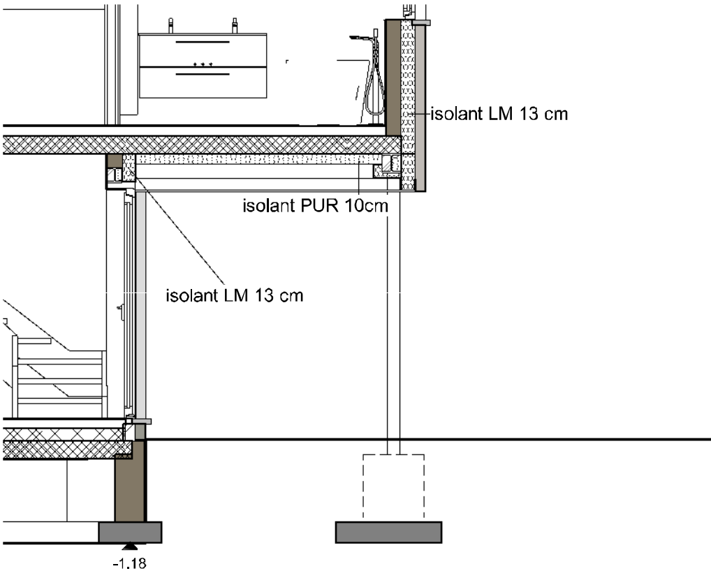
COUPE BB
