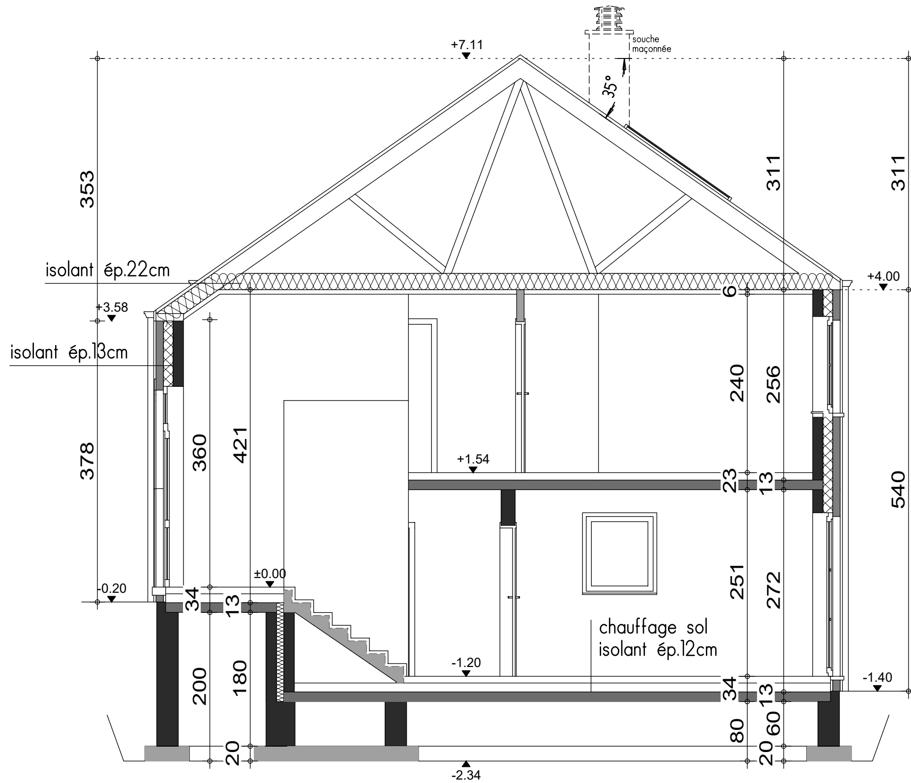
COUPE AA
