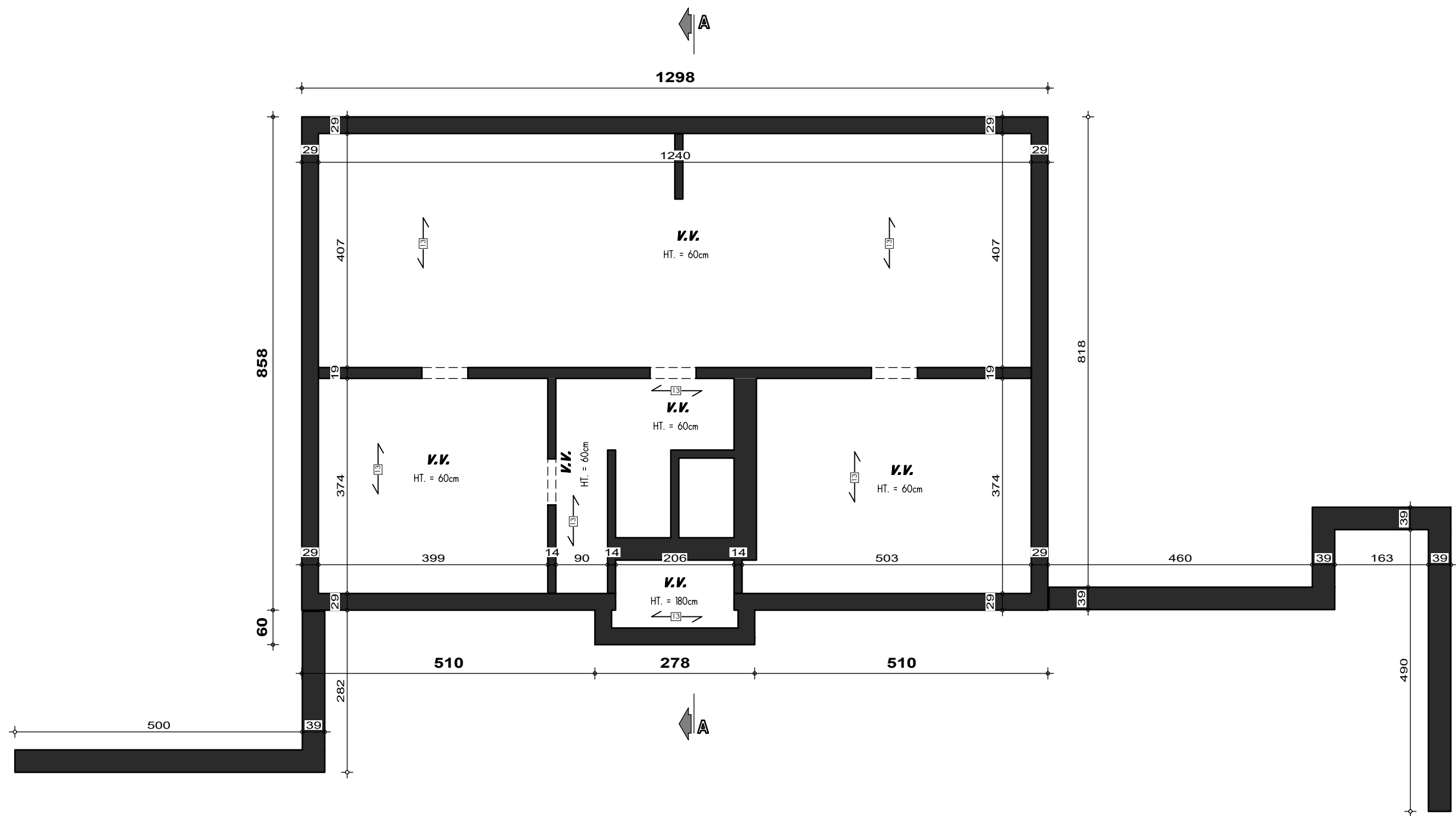
PLAN SOUS-SOL
