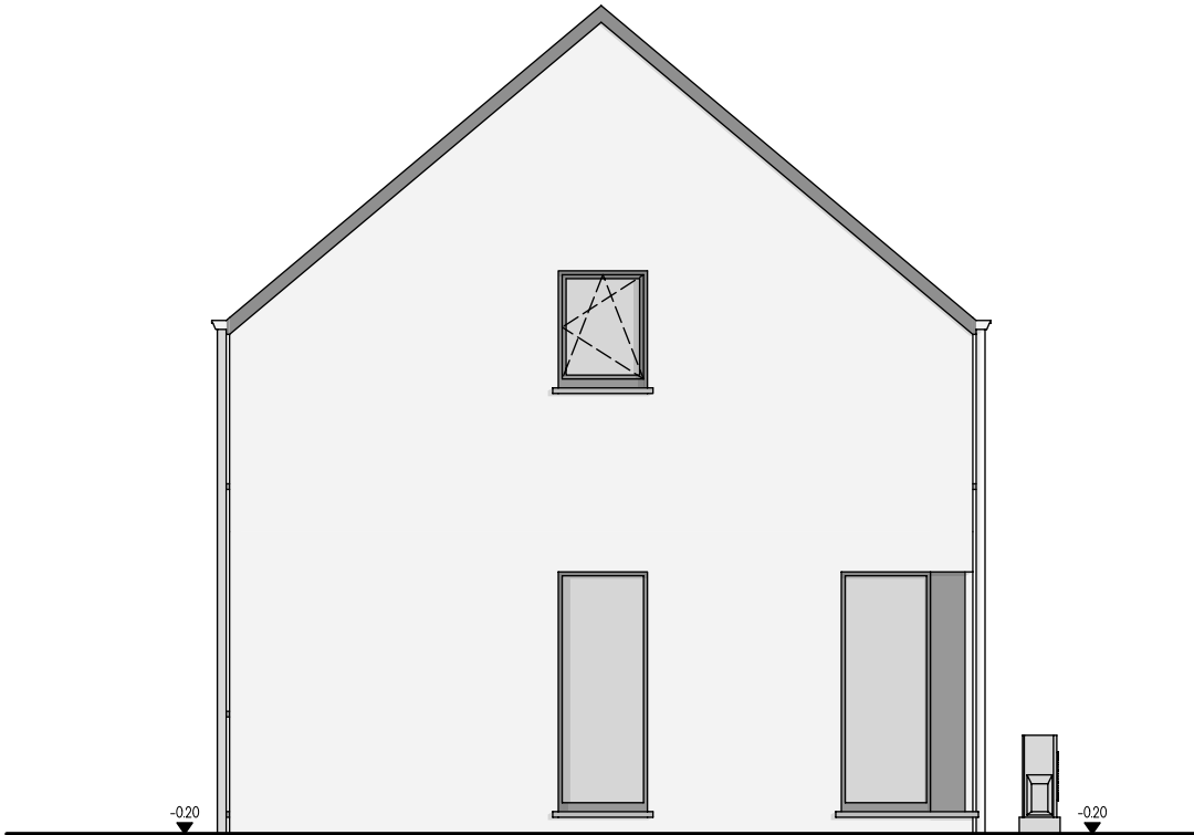
PIGNON DROIT
