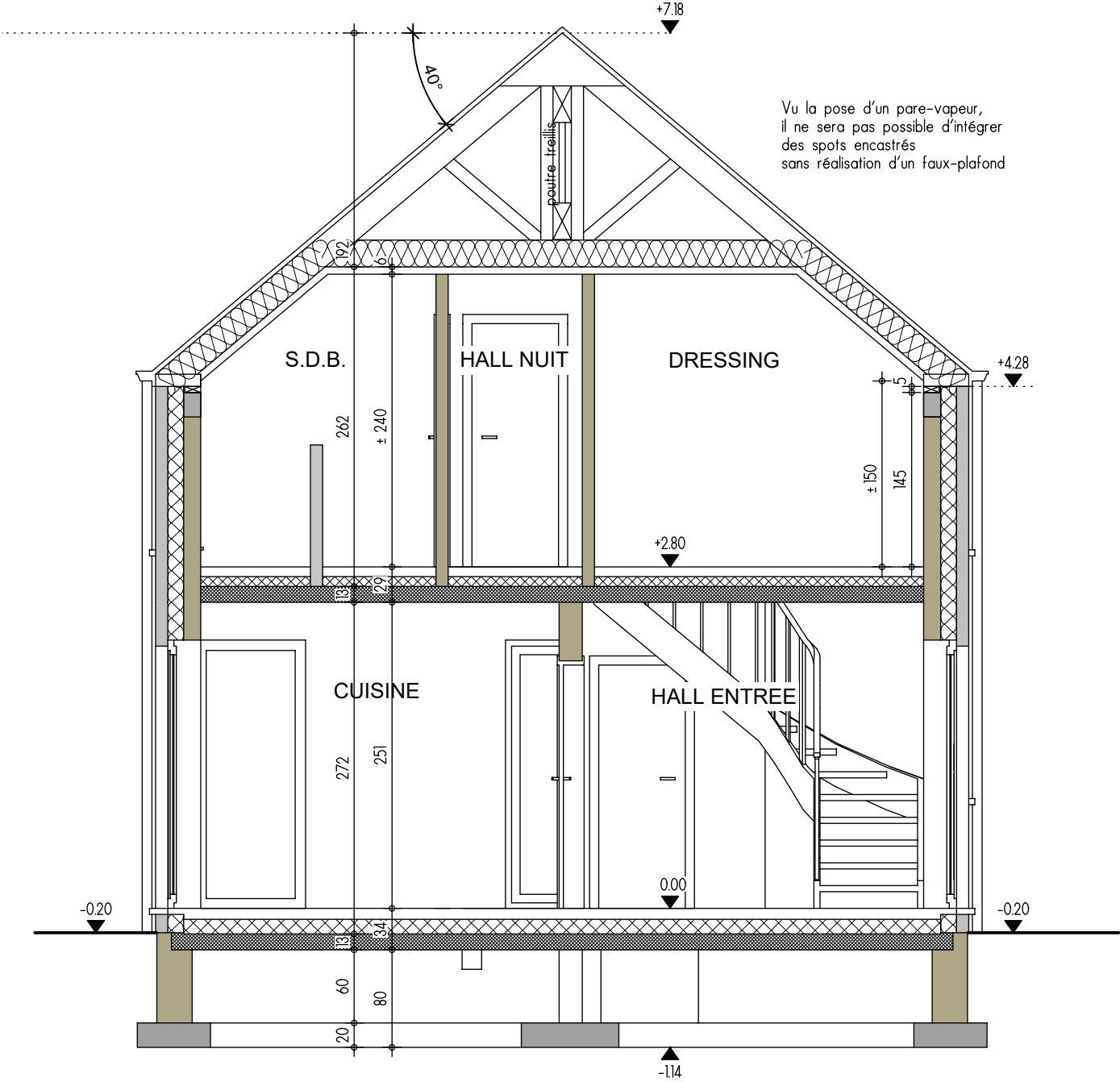
COUPE AA
