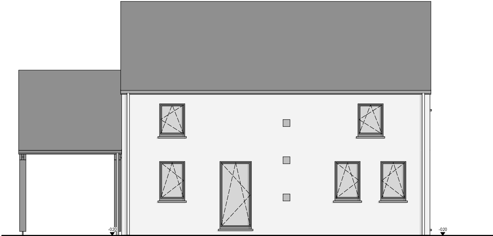
FACADE AVANT
