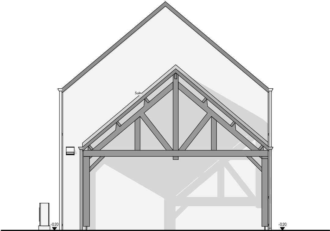
PIGNON GAUCHE
