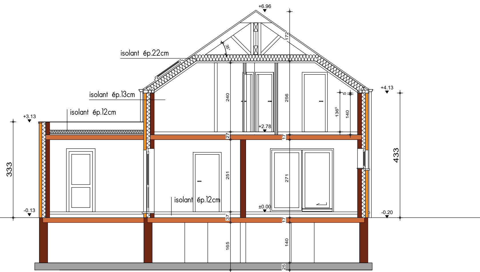
COUPE AA
