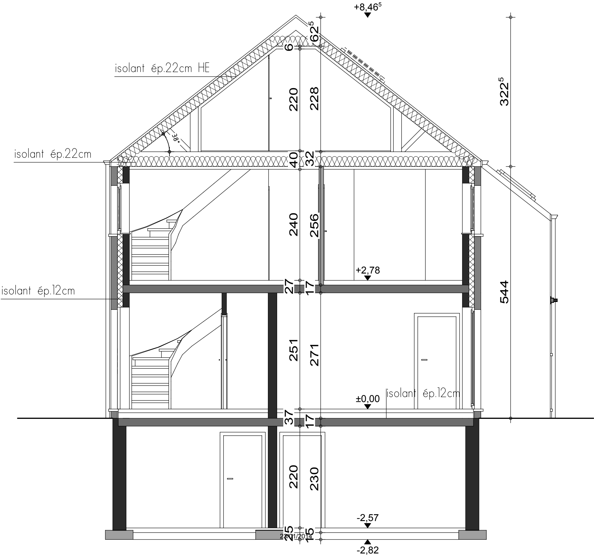
COUPE AA
