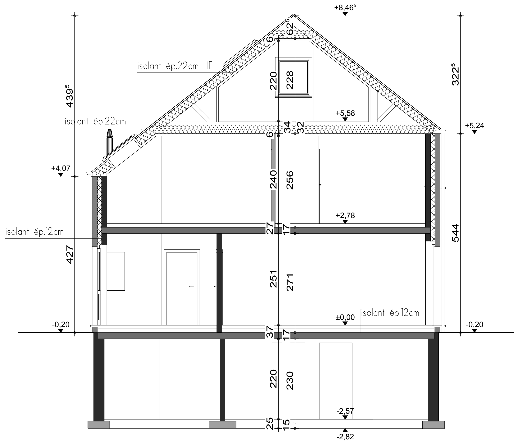
COUPE BB
