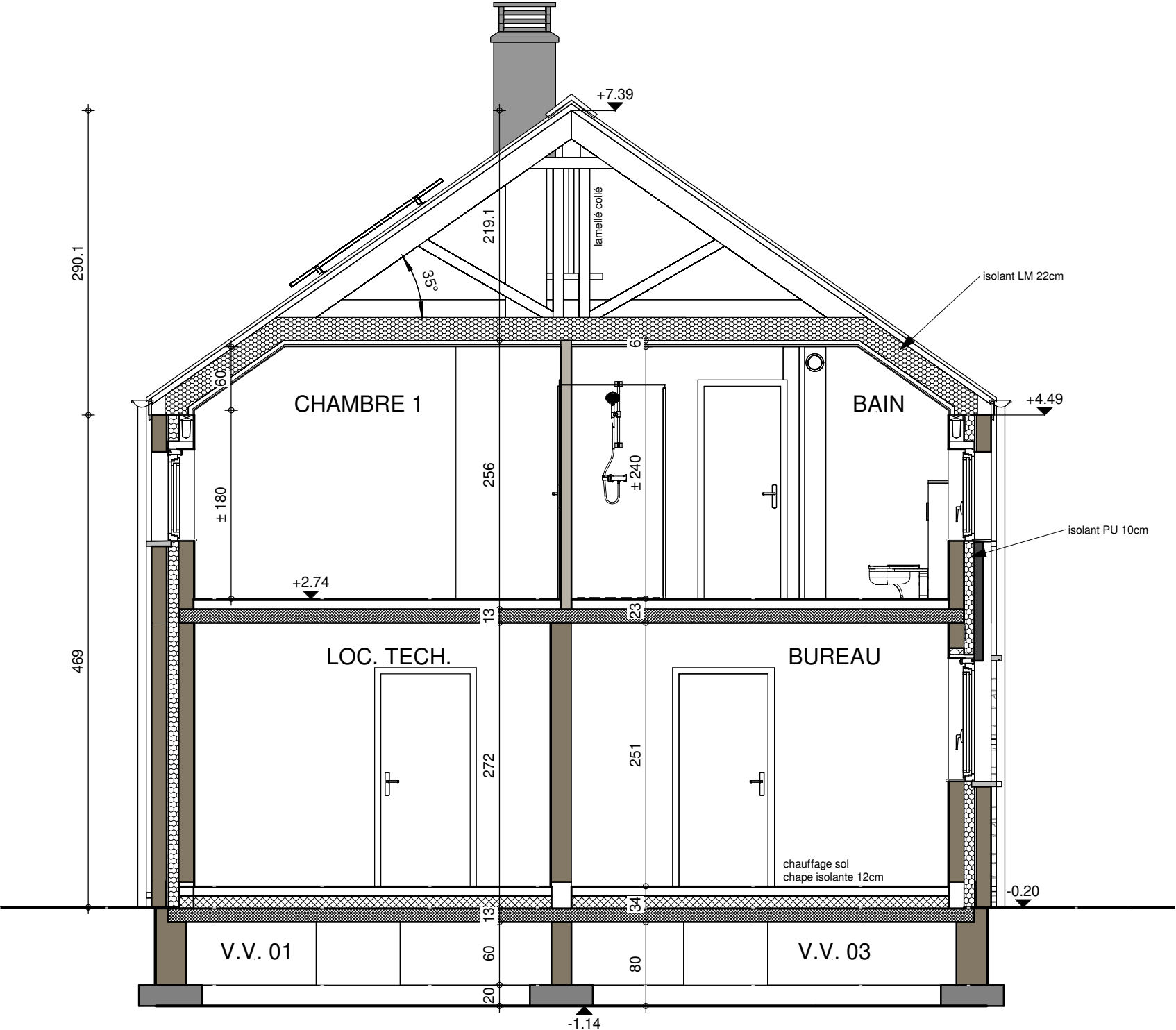
COUPE AA
