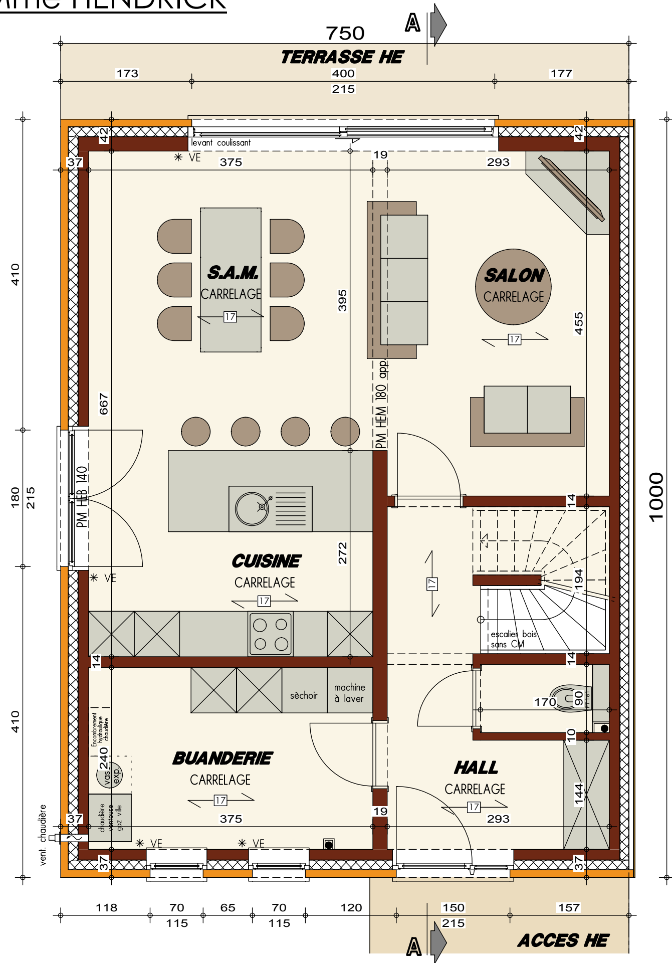
PLAN REZ-DE-CHAUSSEE
