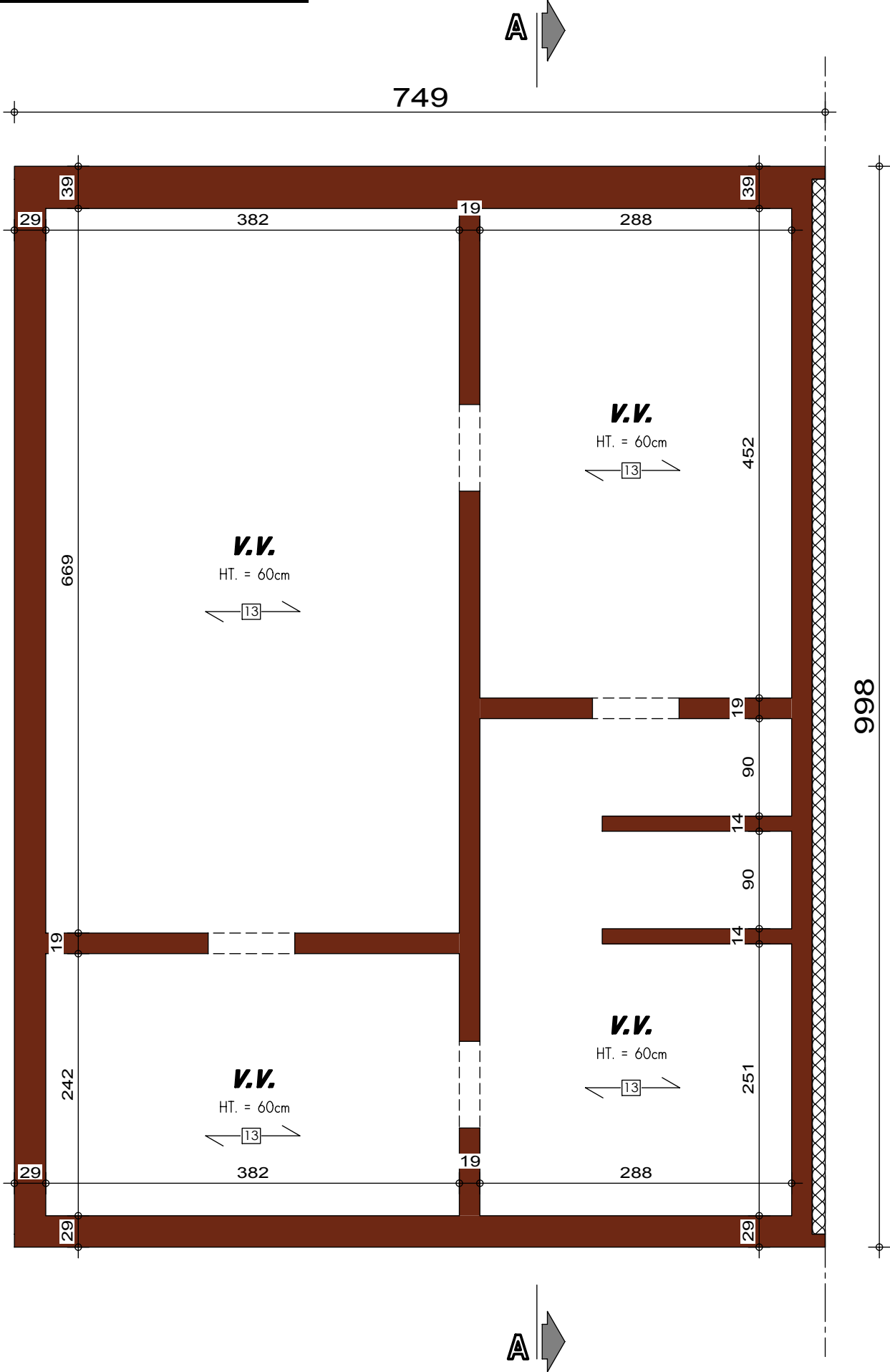
PLAN SOUS-SOL
