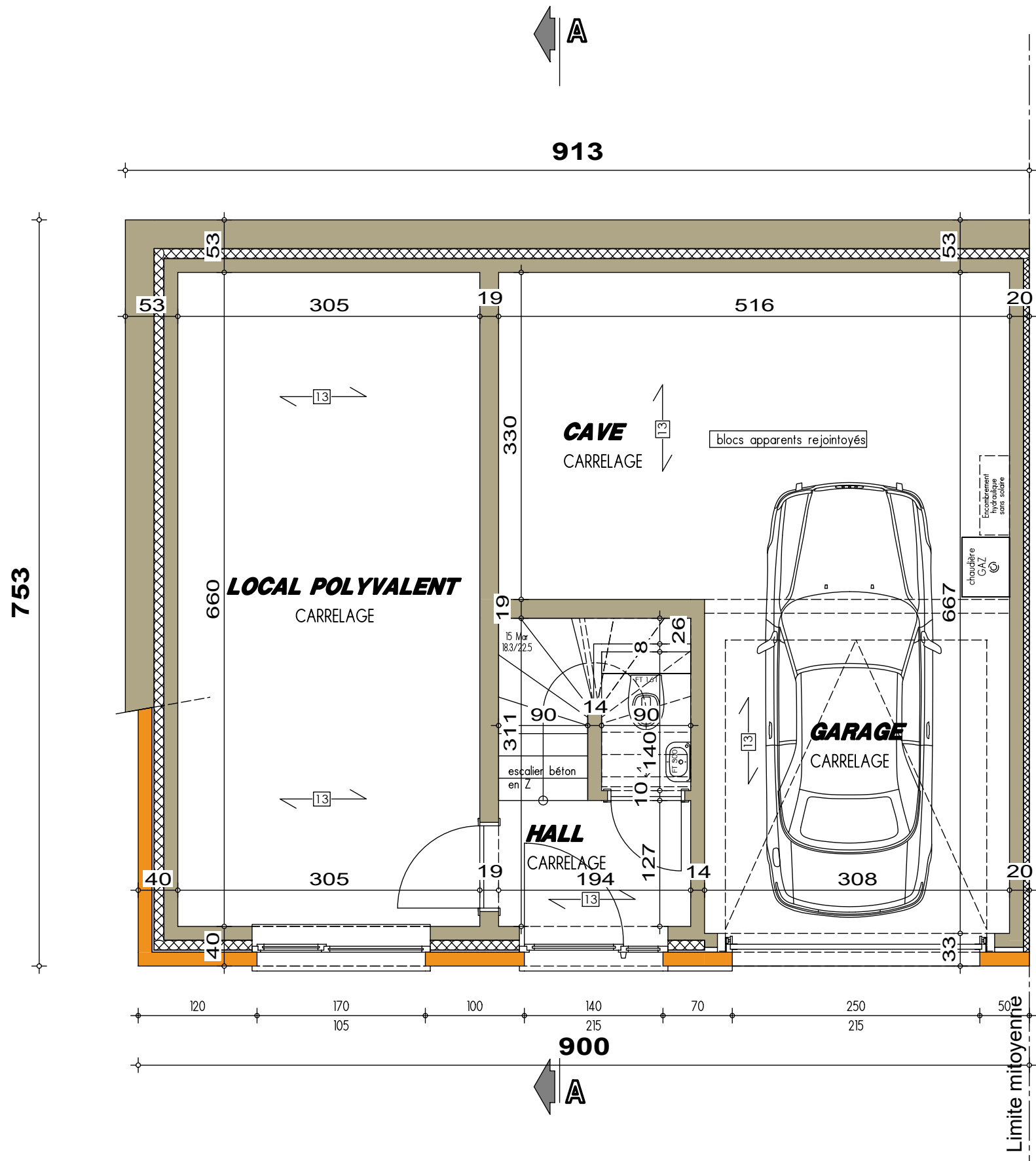
PLAN REZ-DE-CHAUSSEE
