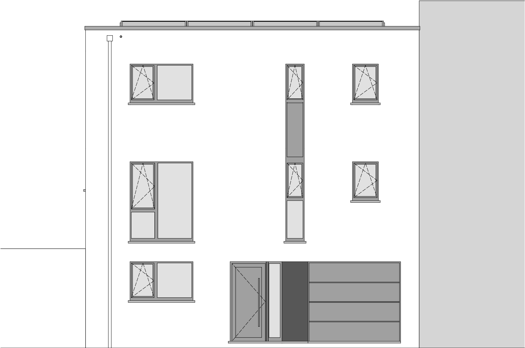
FACADE AVANT
