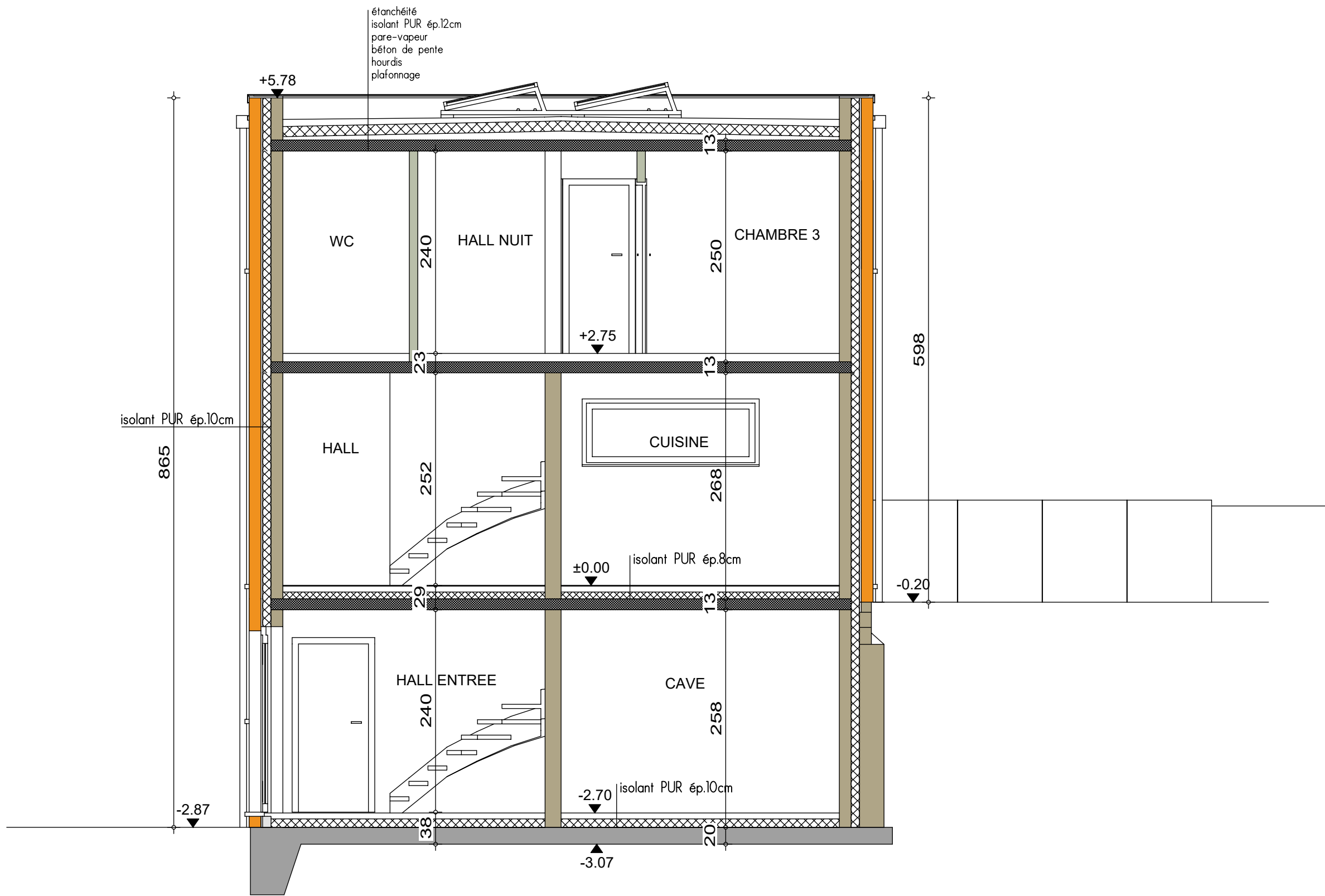
COUPE AA
