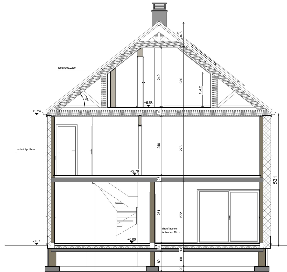
COUPE AA
