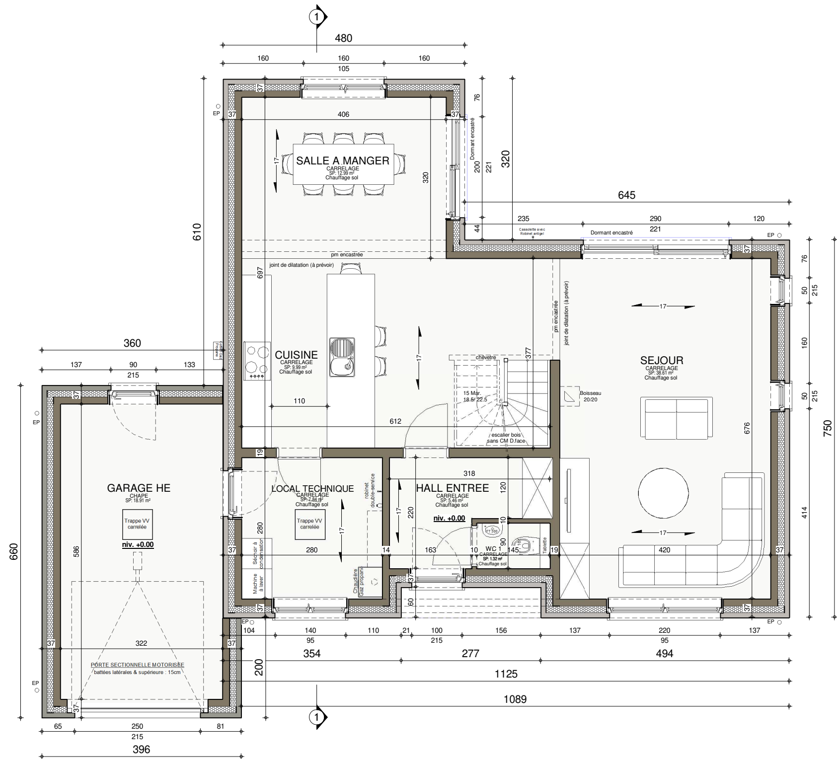
REZ-DE-CHAUSSEE
