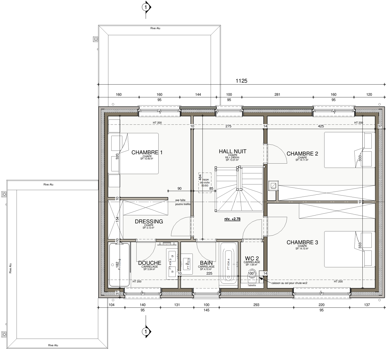
ETAGE
