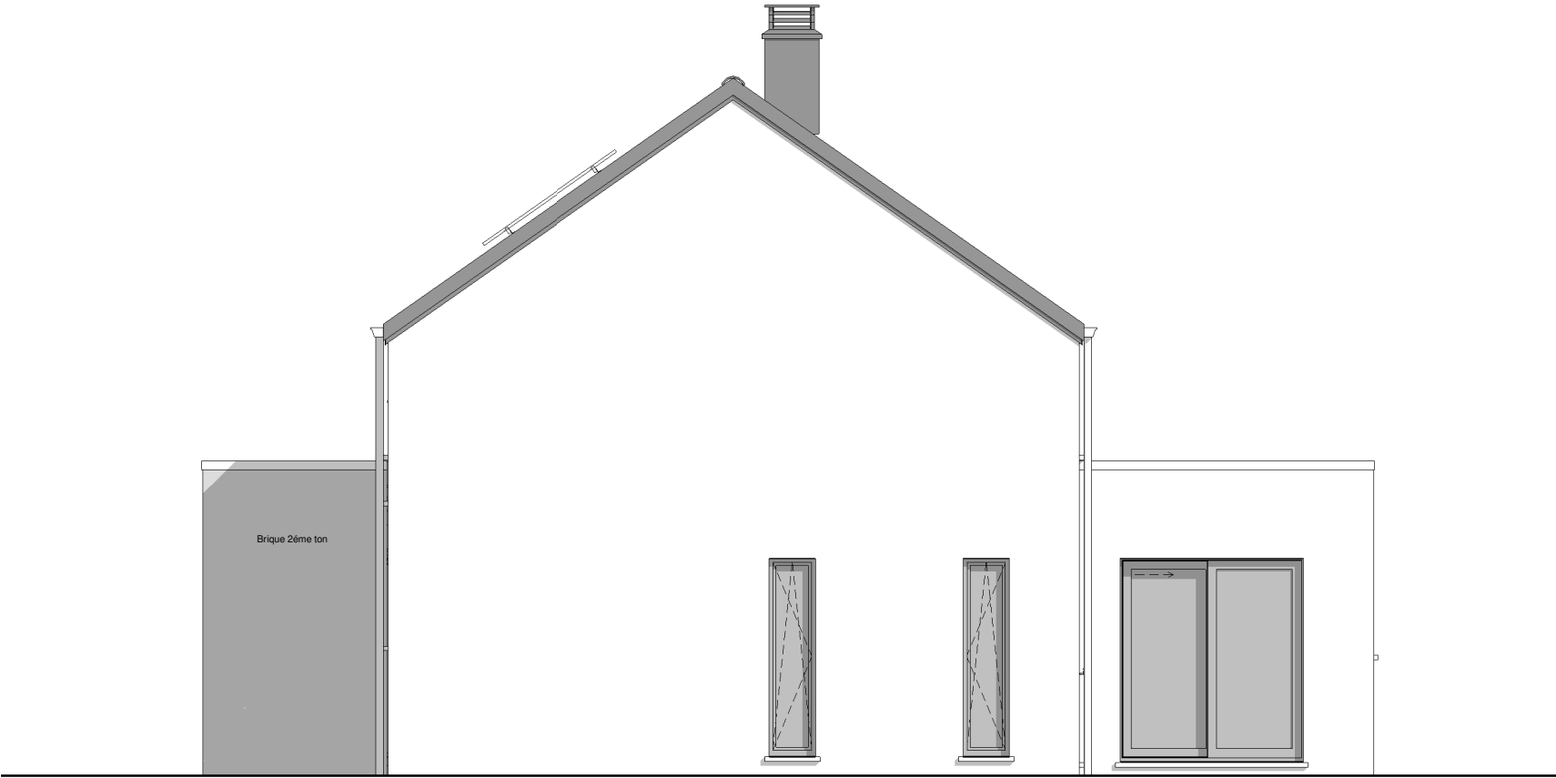
PIGNON DROIT
