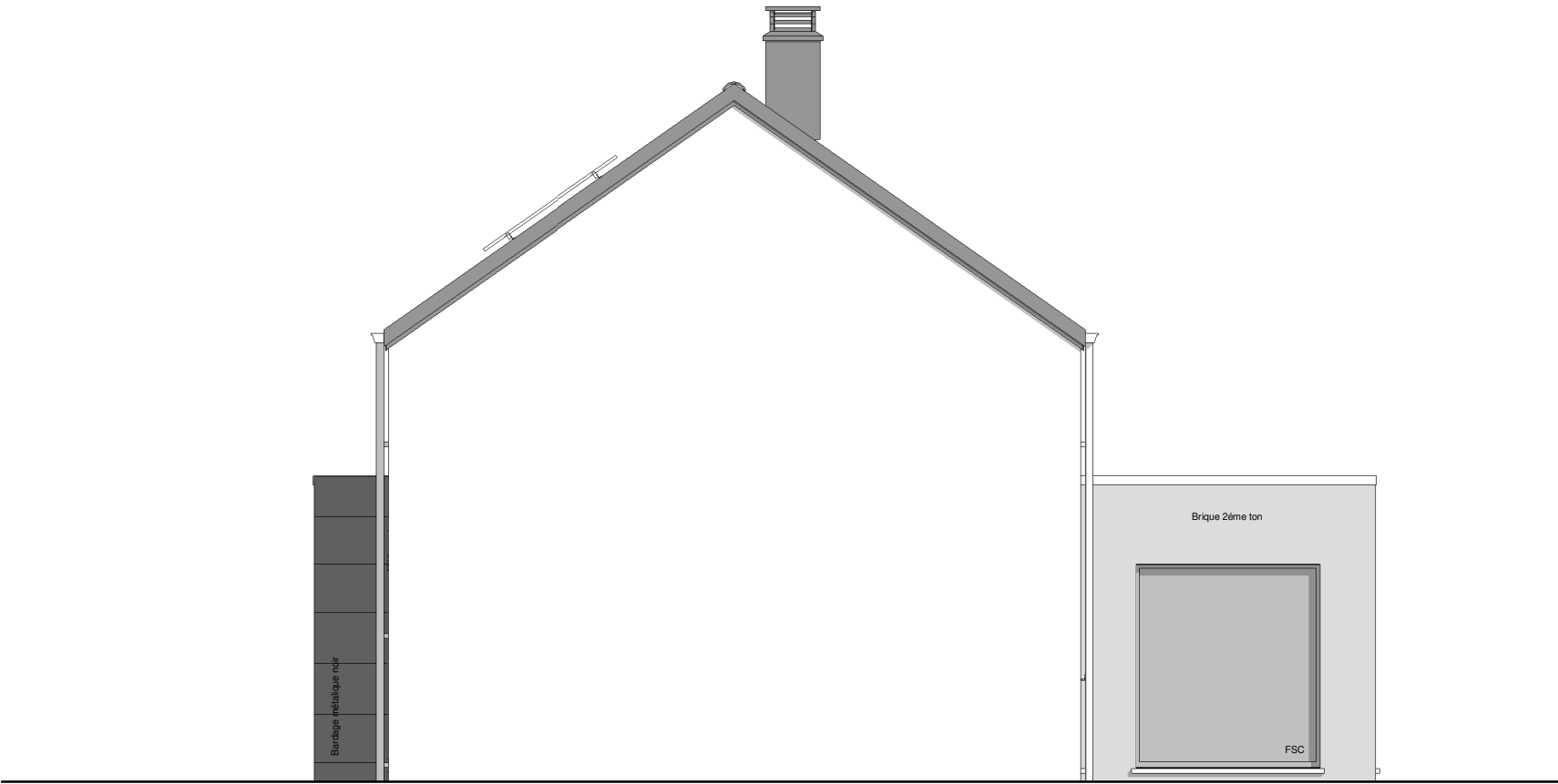
PIGNON DROIT
