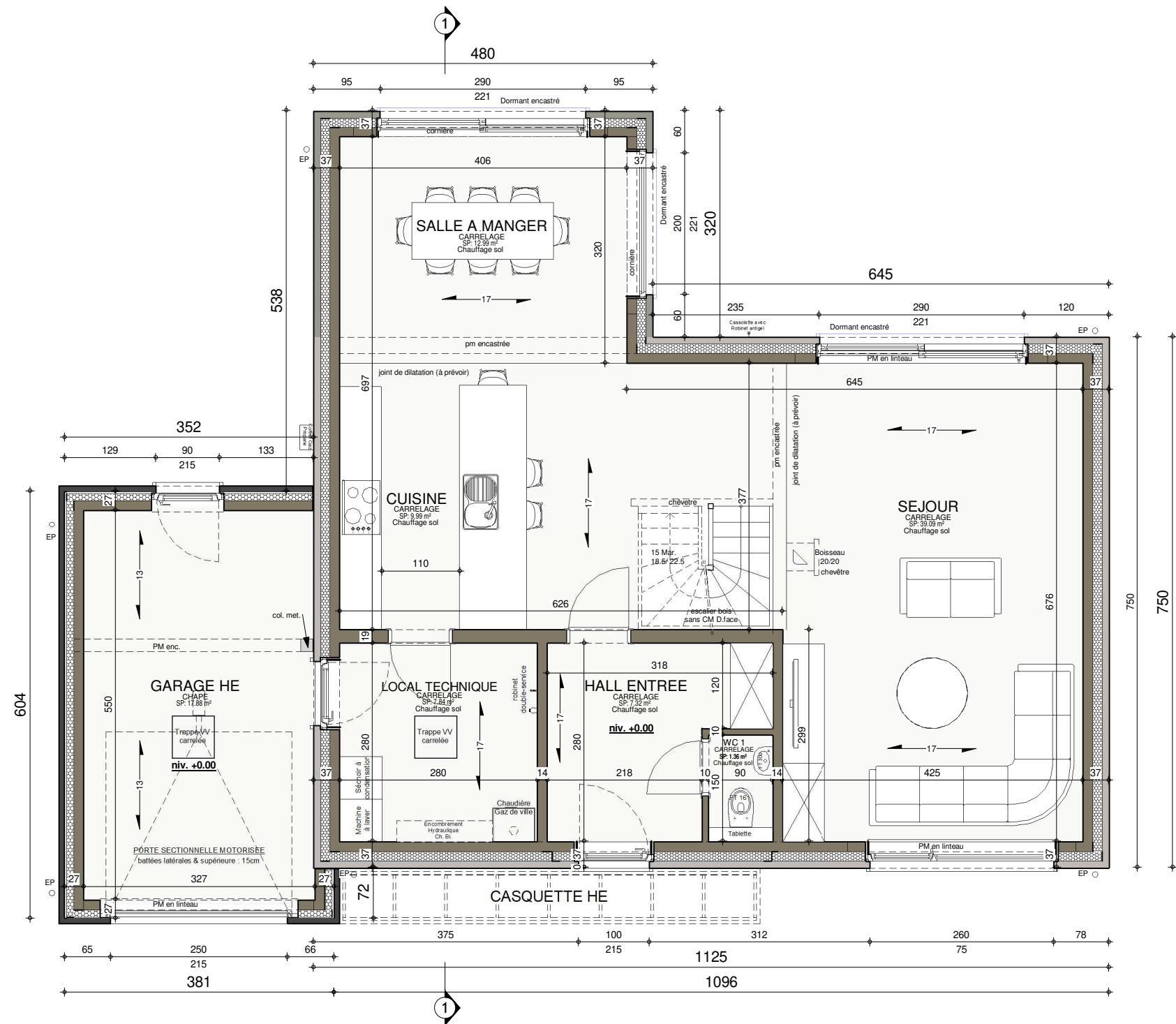
REZ-DE-CHAUSSEE
