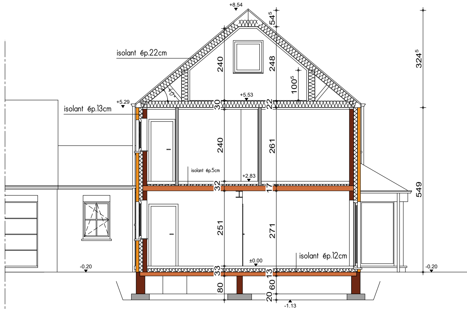
COUPE AA
