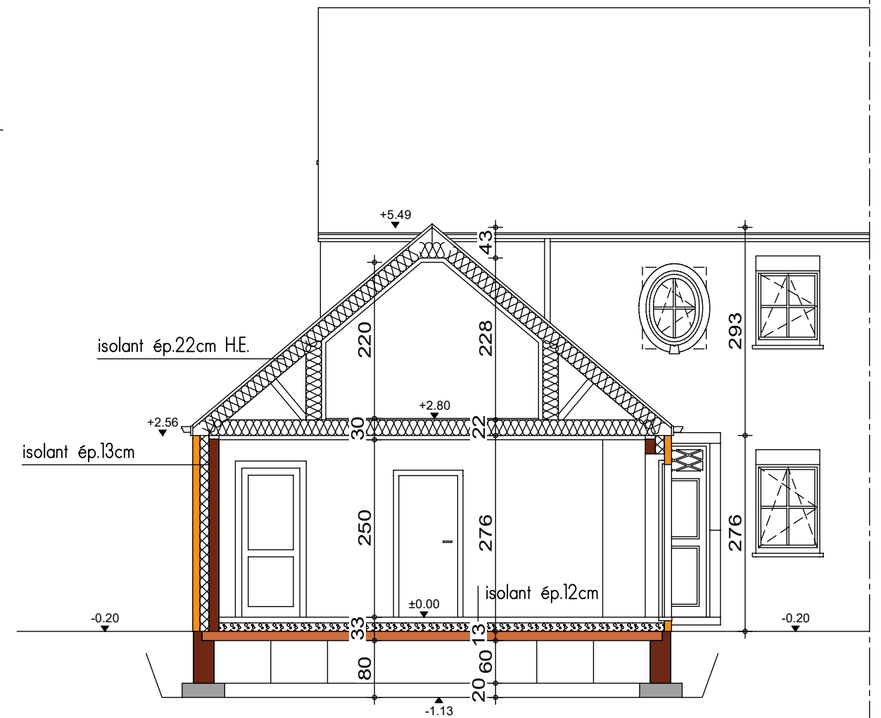
COUPE BB
