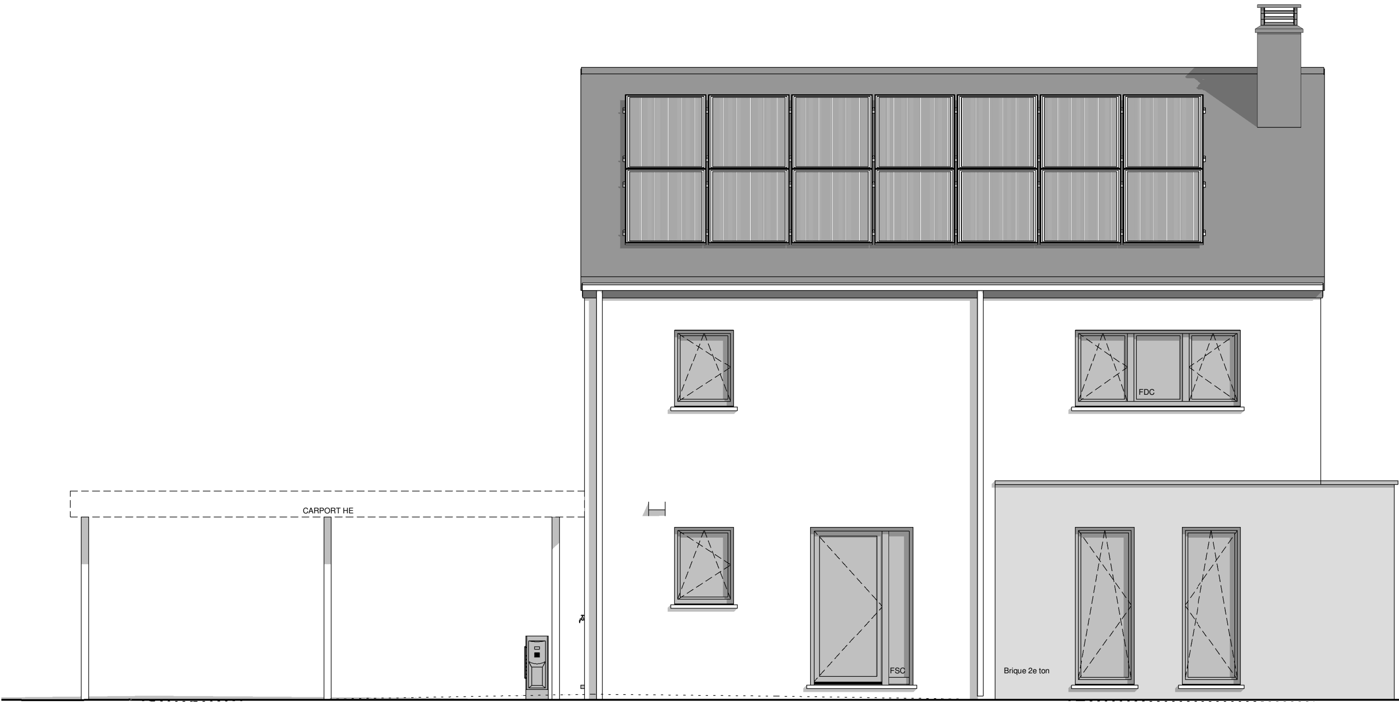
FACADE AVANT
