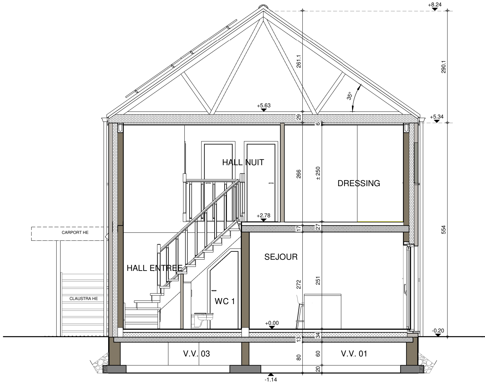
COUPE AA
