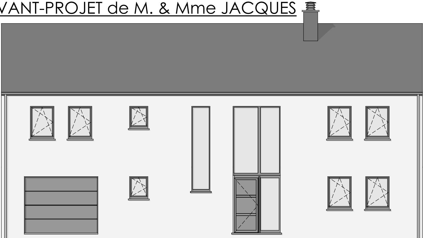
FACADE AVANT
