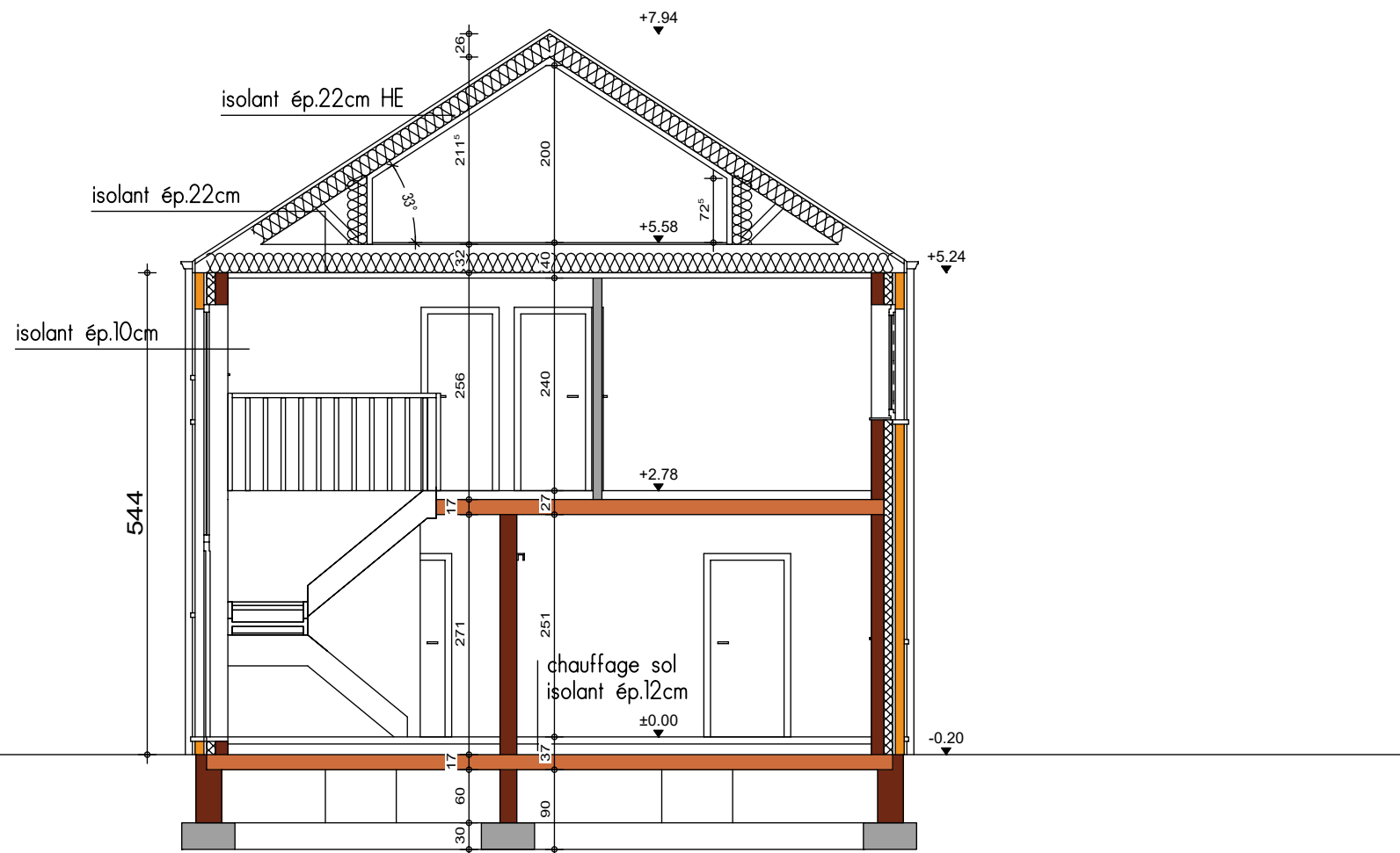
COUPE AA
