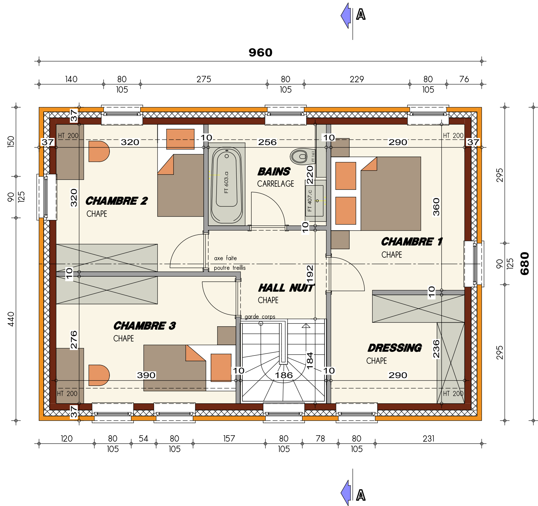
PLAN ETAGE
