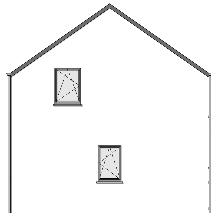
PIGNON GAUCHE
