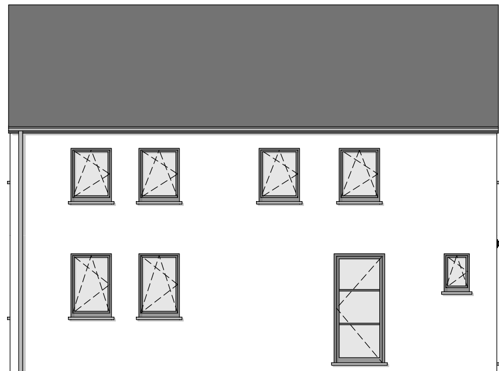
FACADE AVANT
