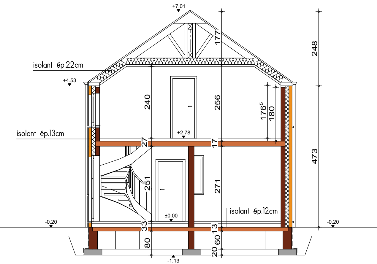
COUPE AA
