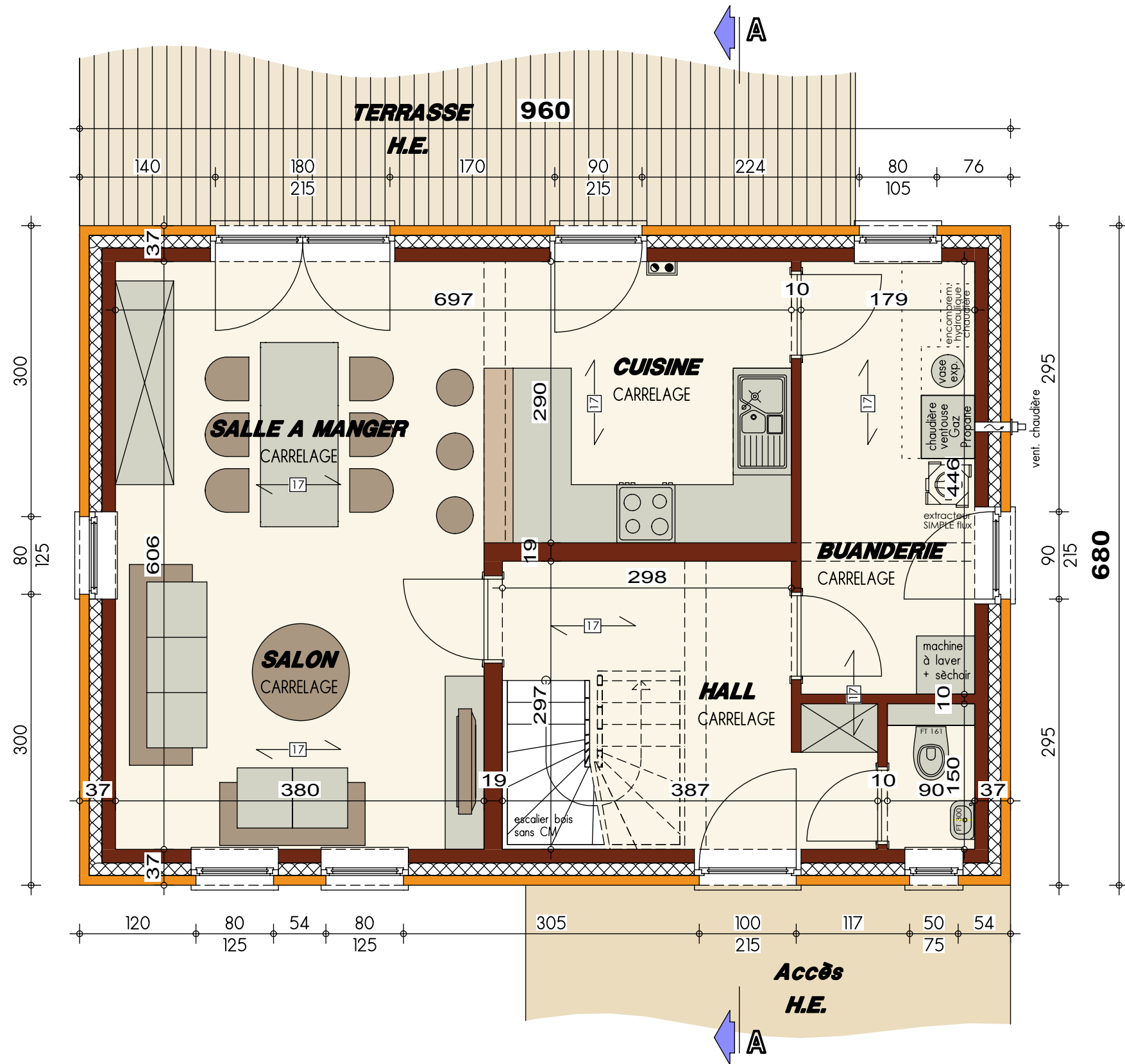
PLAN REZ-DE-CHAUSSEE
