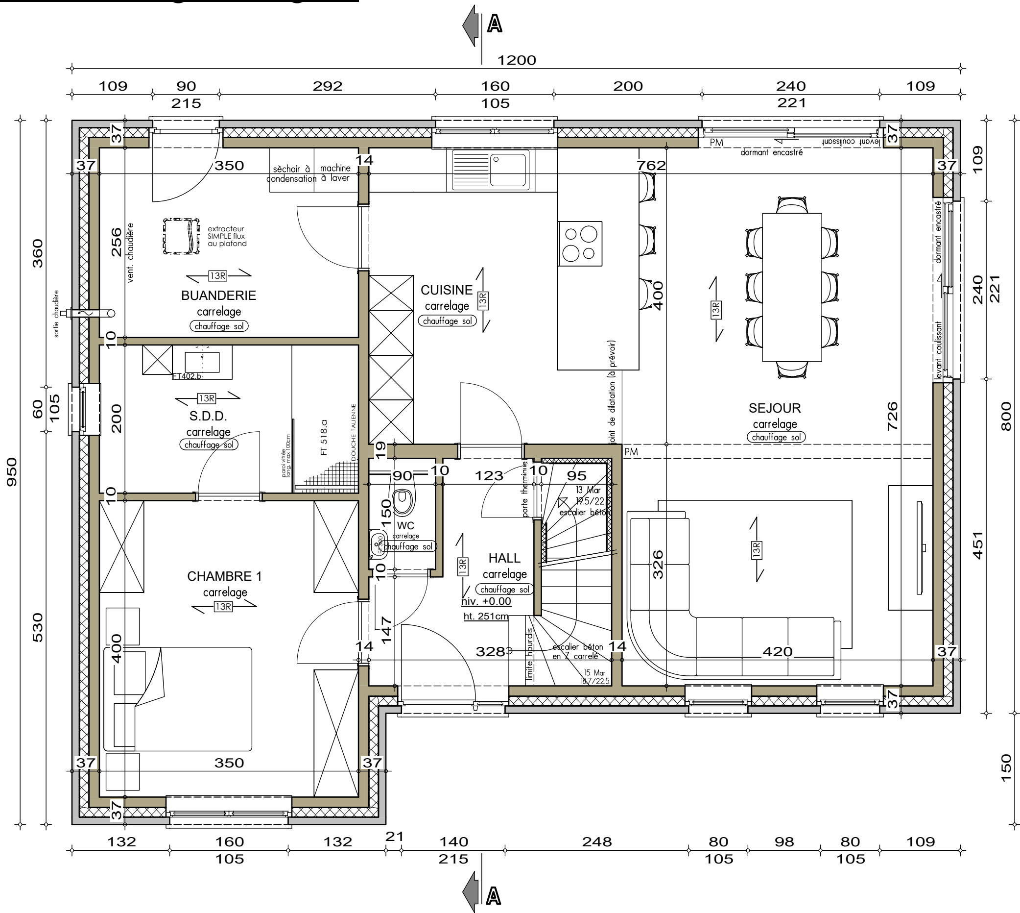
PLAN REZ-DE-CHAUSSEE
