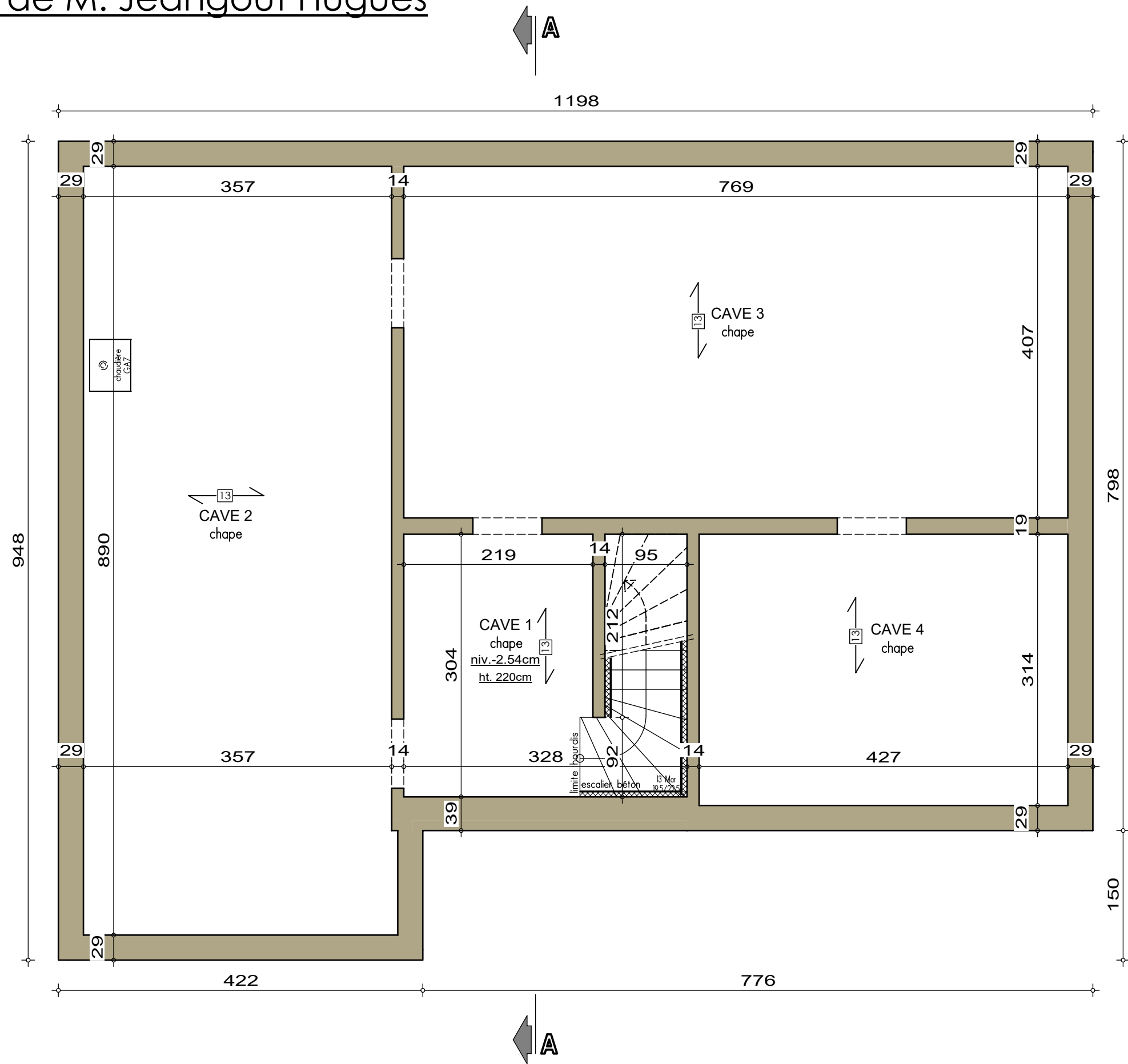
PLAN SOUS-SOL
