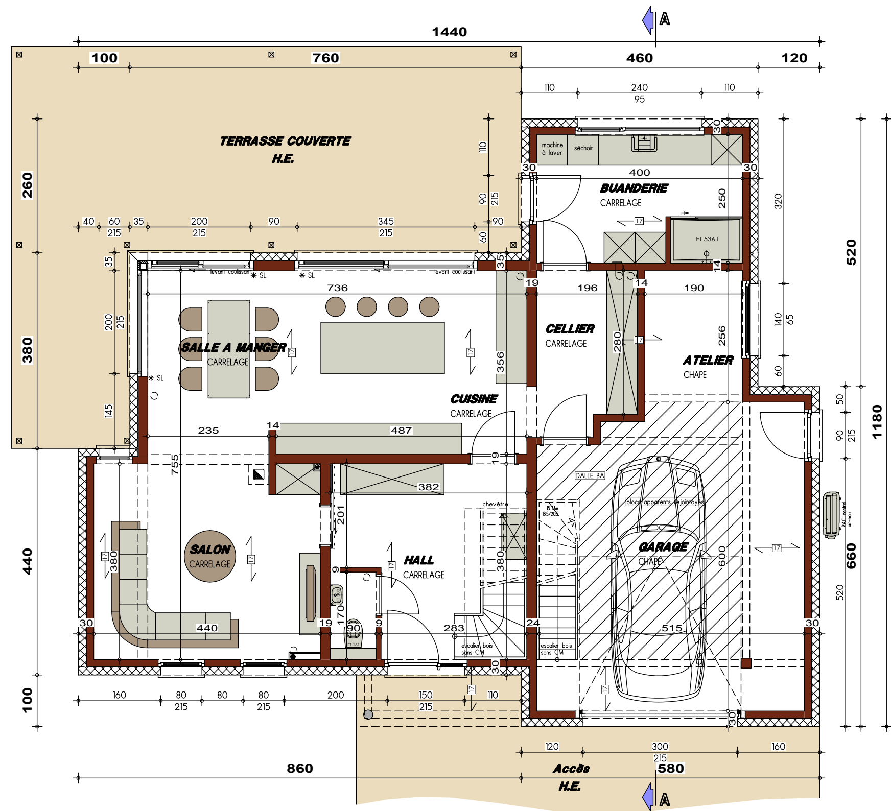
PLAN REZ-DE-CHAUSSEE
