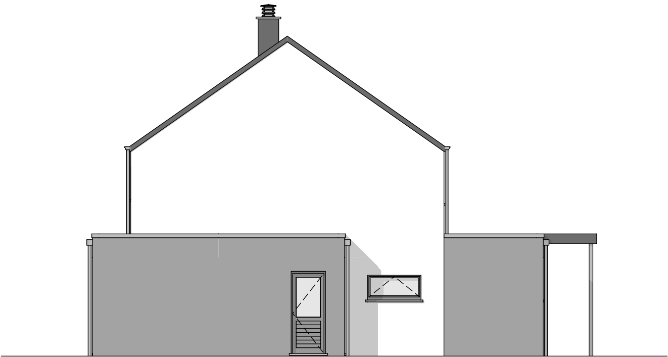
PIGNON DROIT
