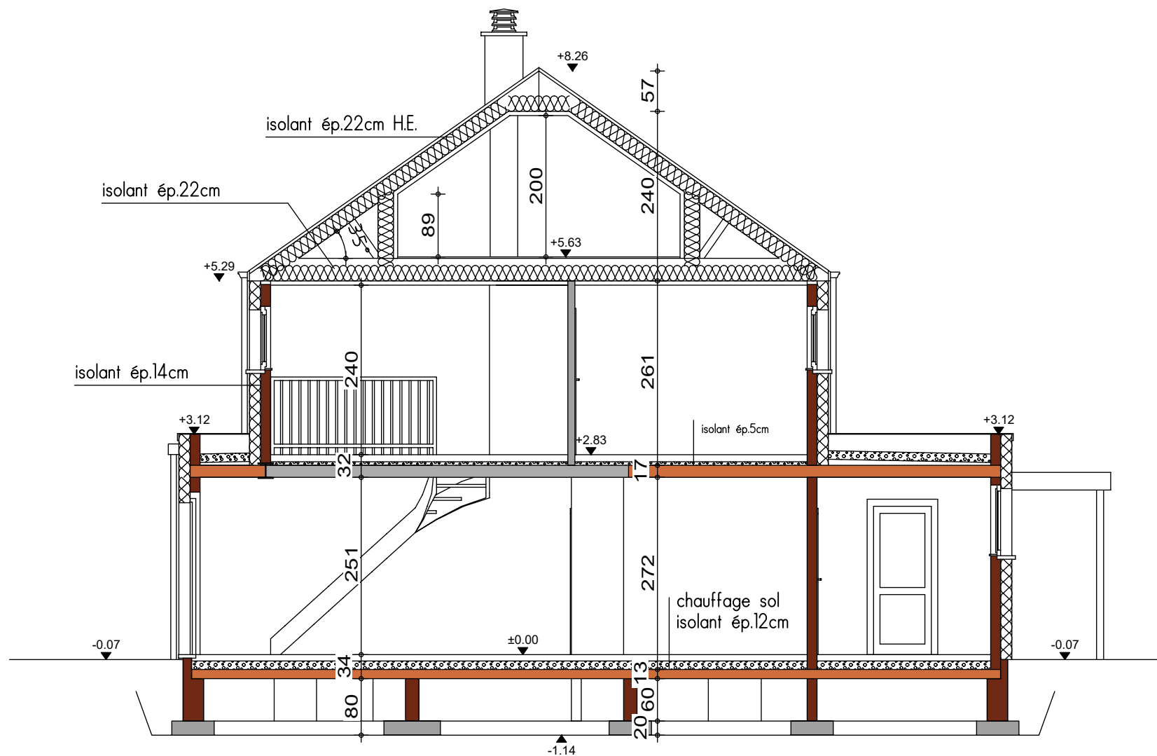
COUPE AA
