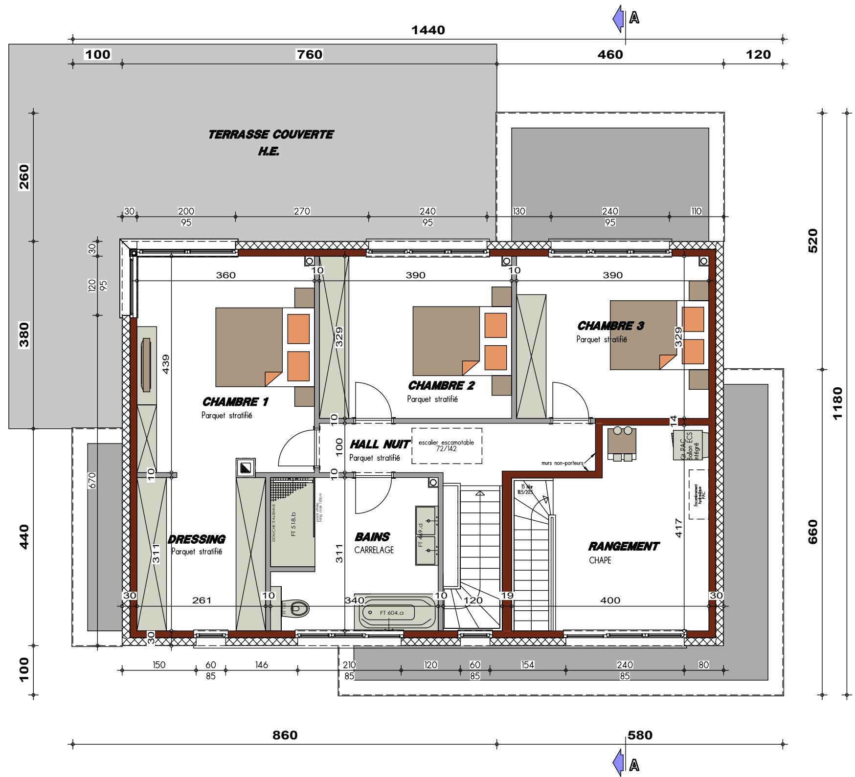
PLAN ETAGE
