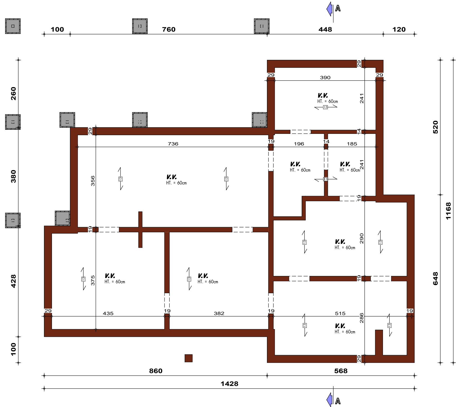
PLAN SOUS-SOL
