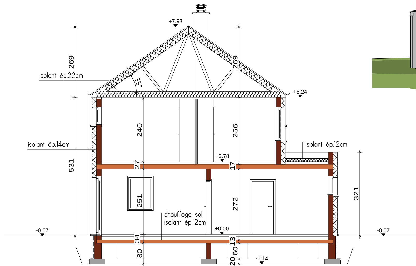
COUPE AA
