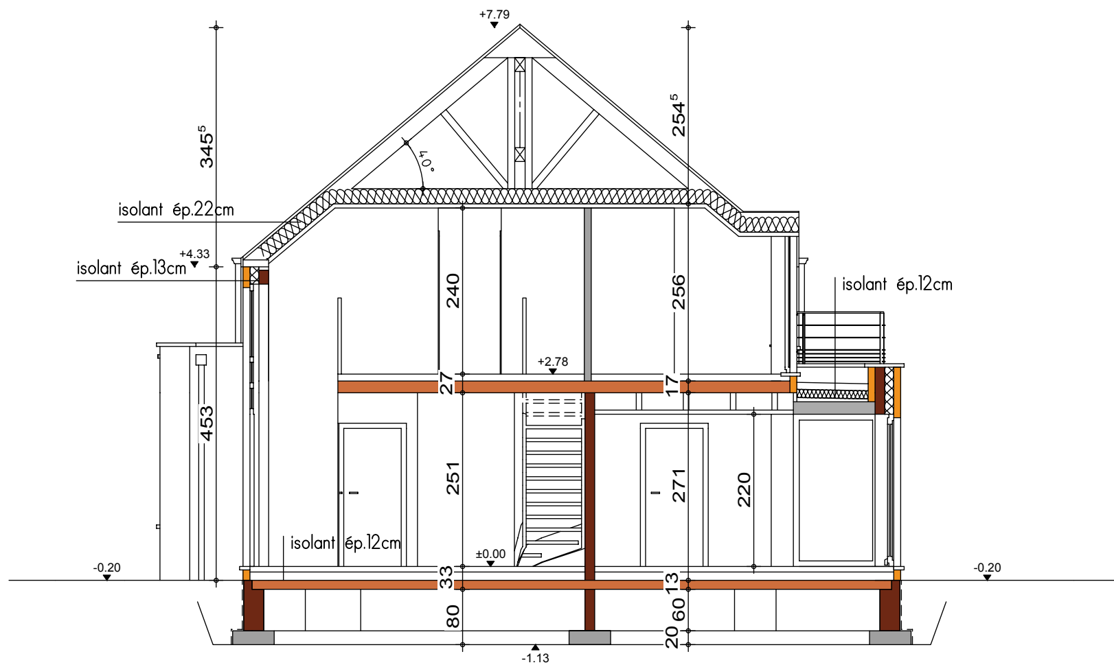
COUPE AA
