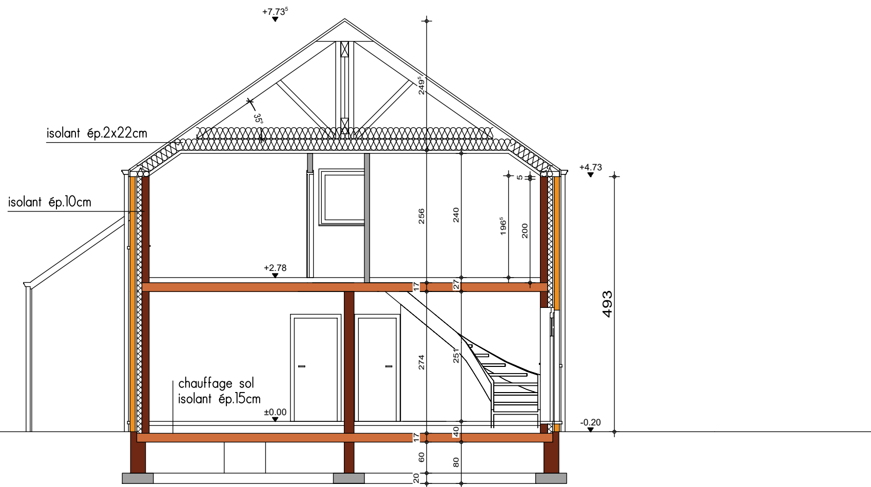
COUPE AA
