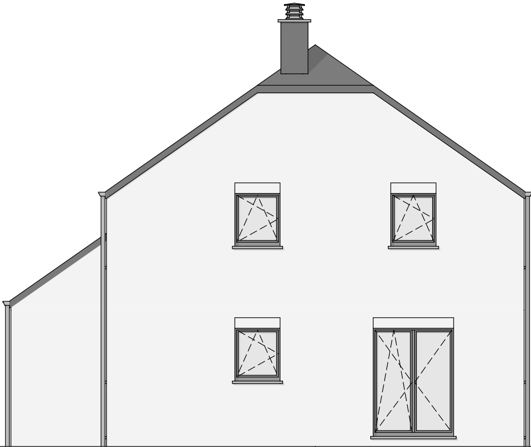
PIGNON GAUCHE
