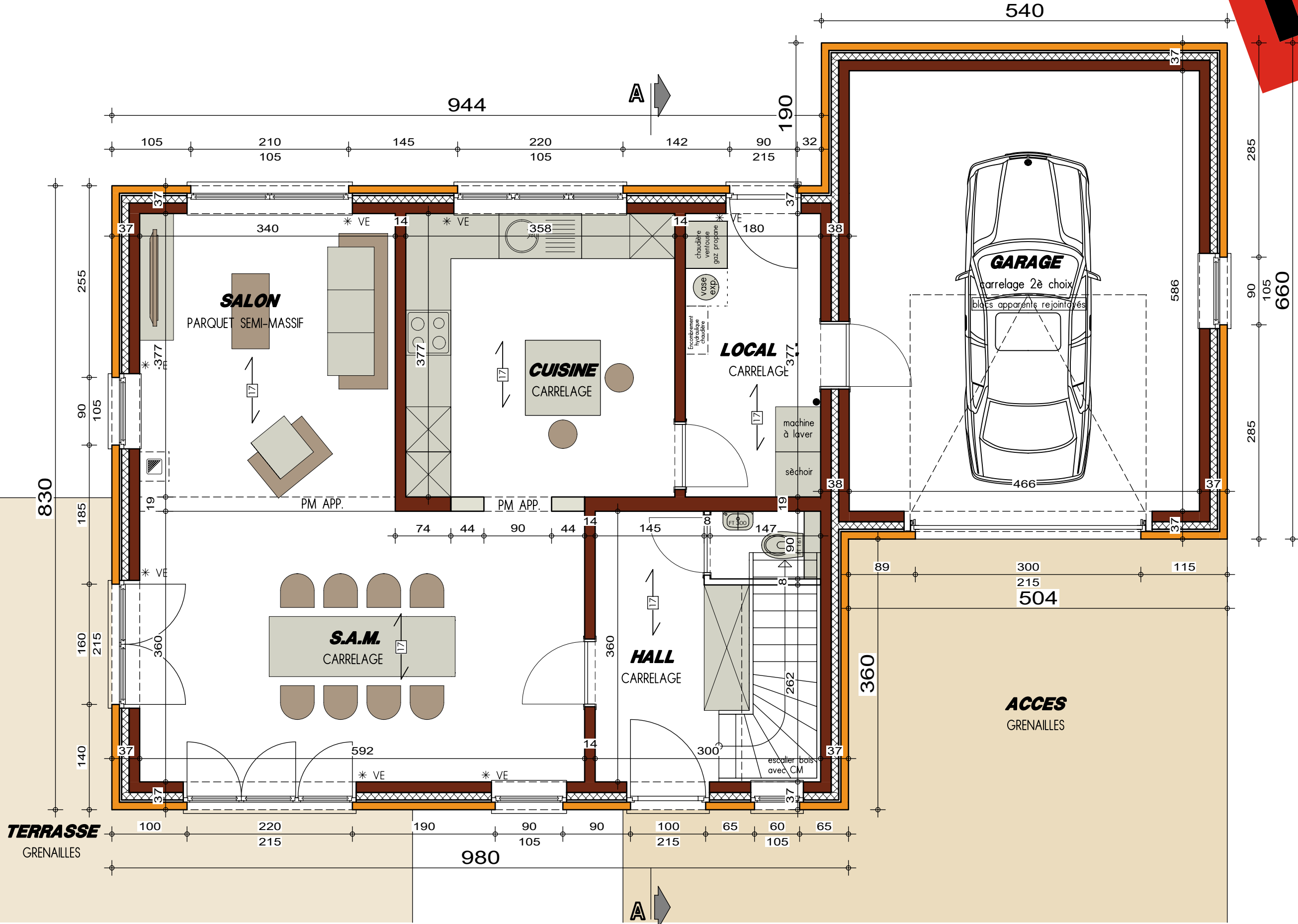
PLAN REZ-DE-CHAUSSEE
