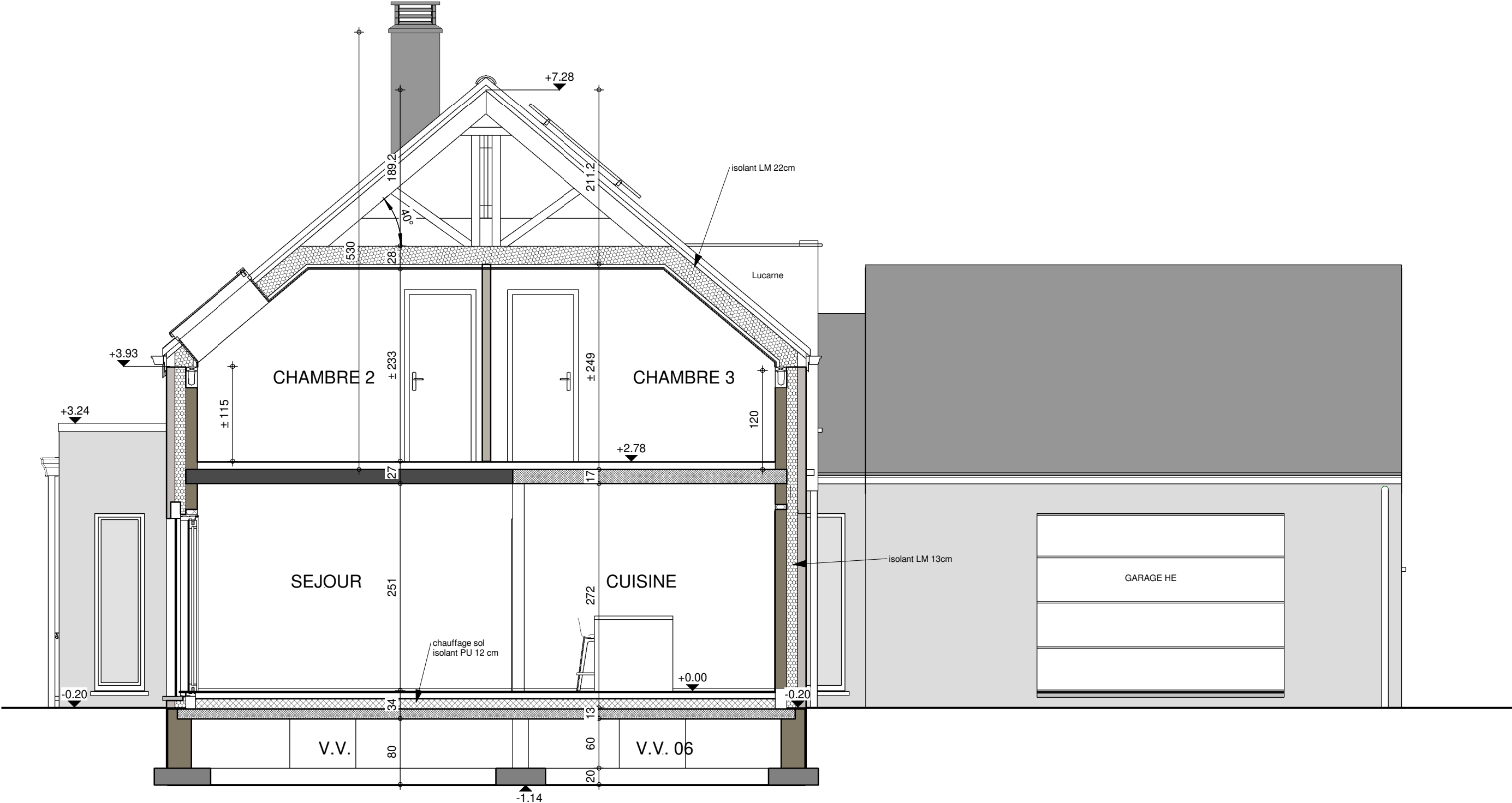
COUPE AA
