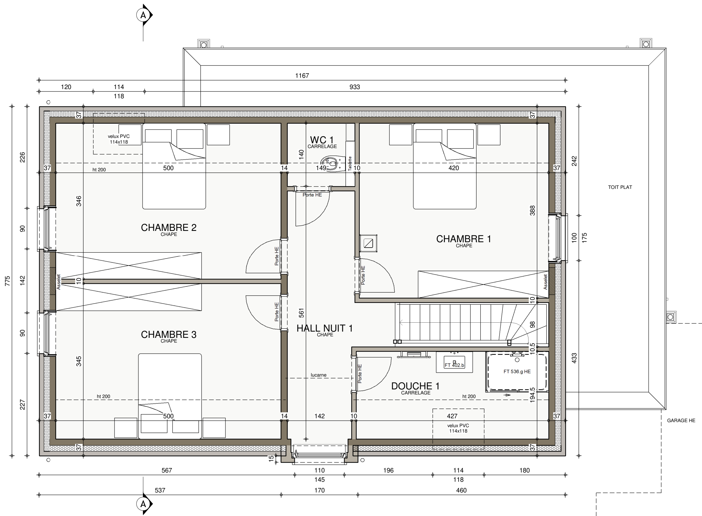
ETAGE
