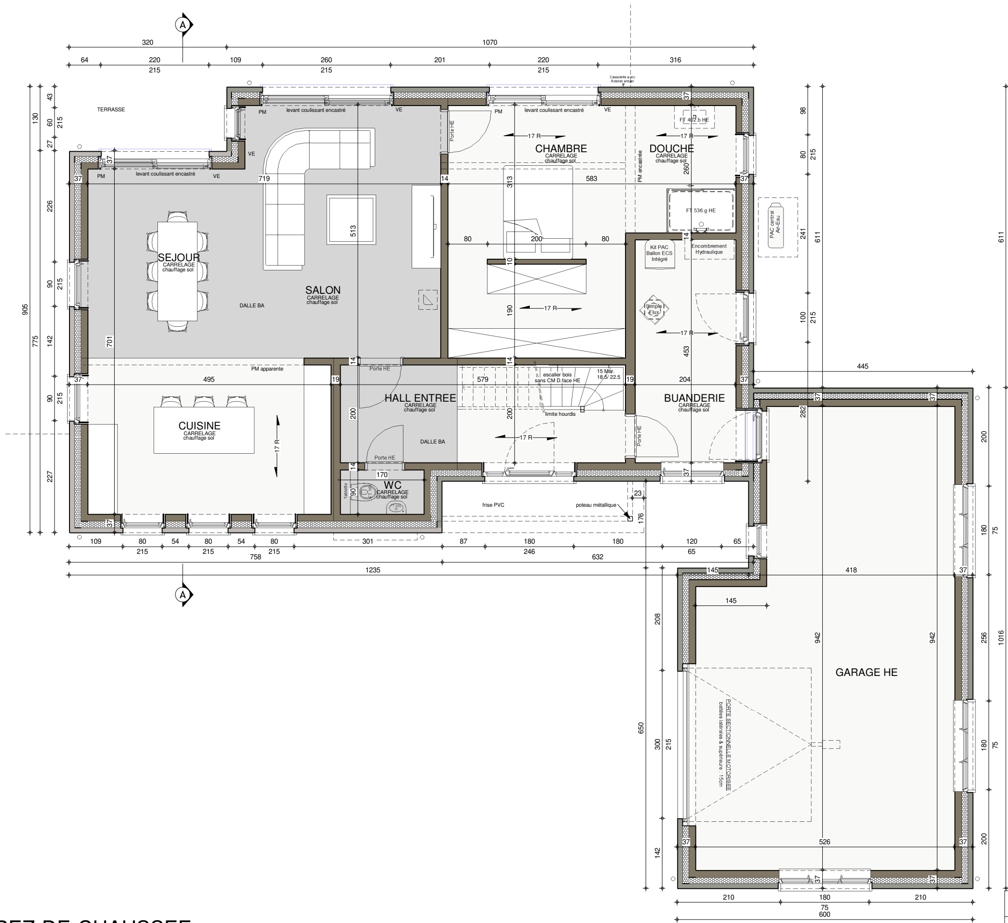
REZ-DE-CHAUSSEE
