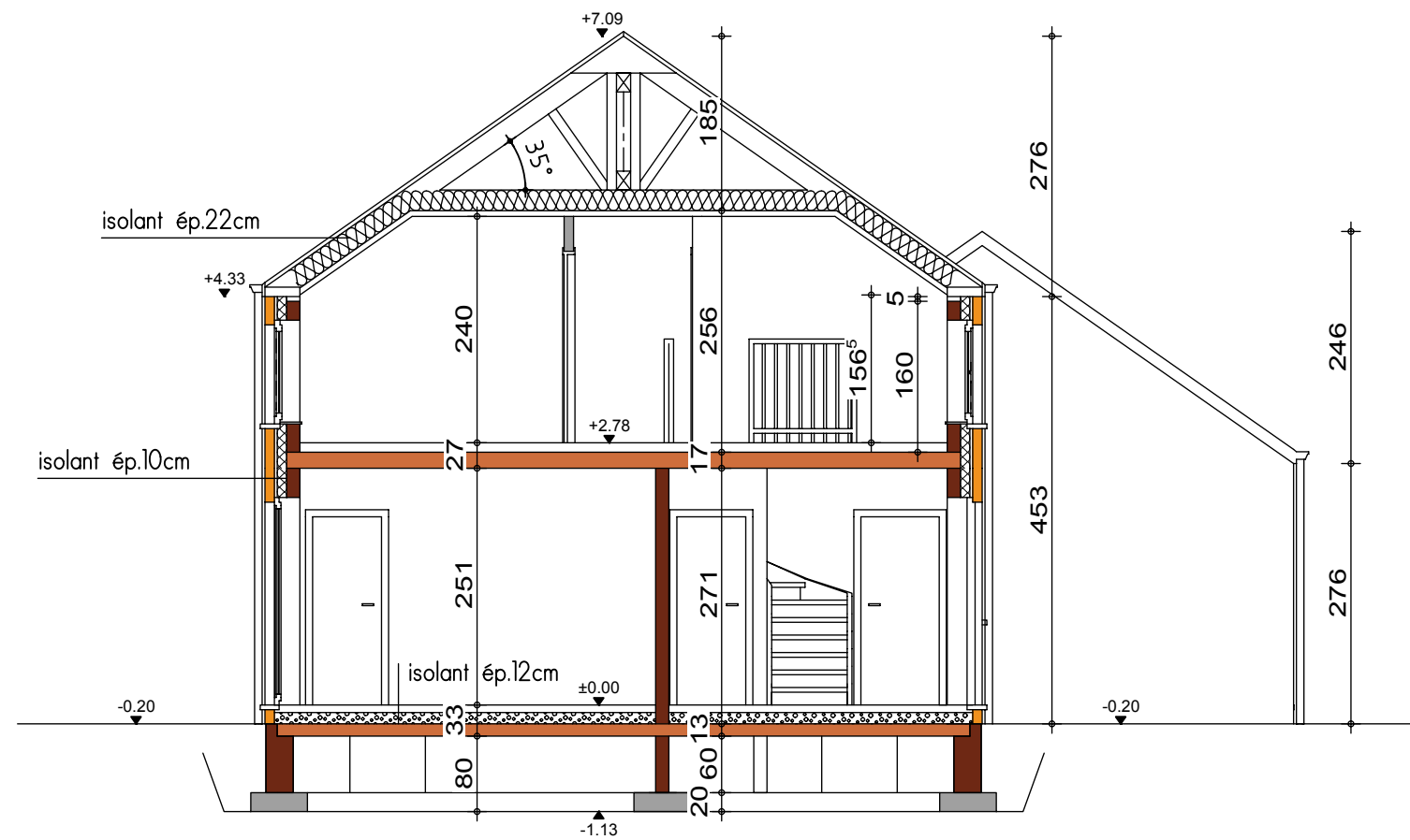
COUPE AA
