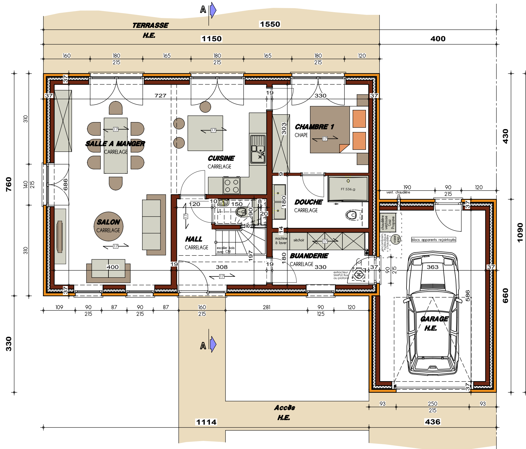
PLAN REZ-DE-CHAUSSEE
