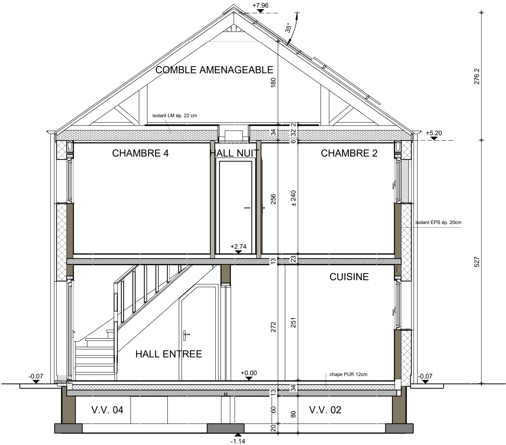
COUPE AA
