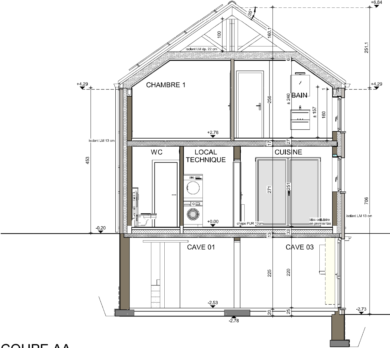
COUPE AA
