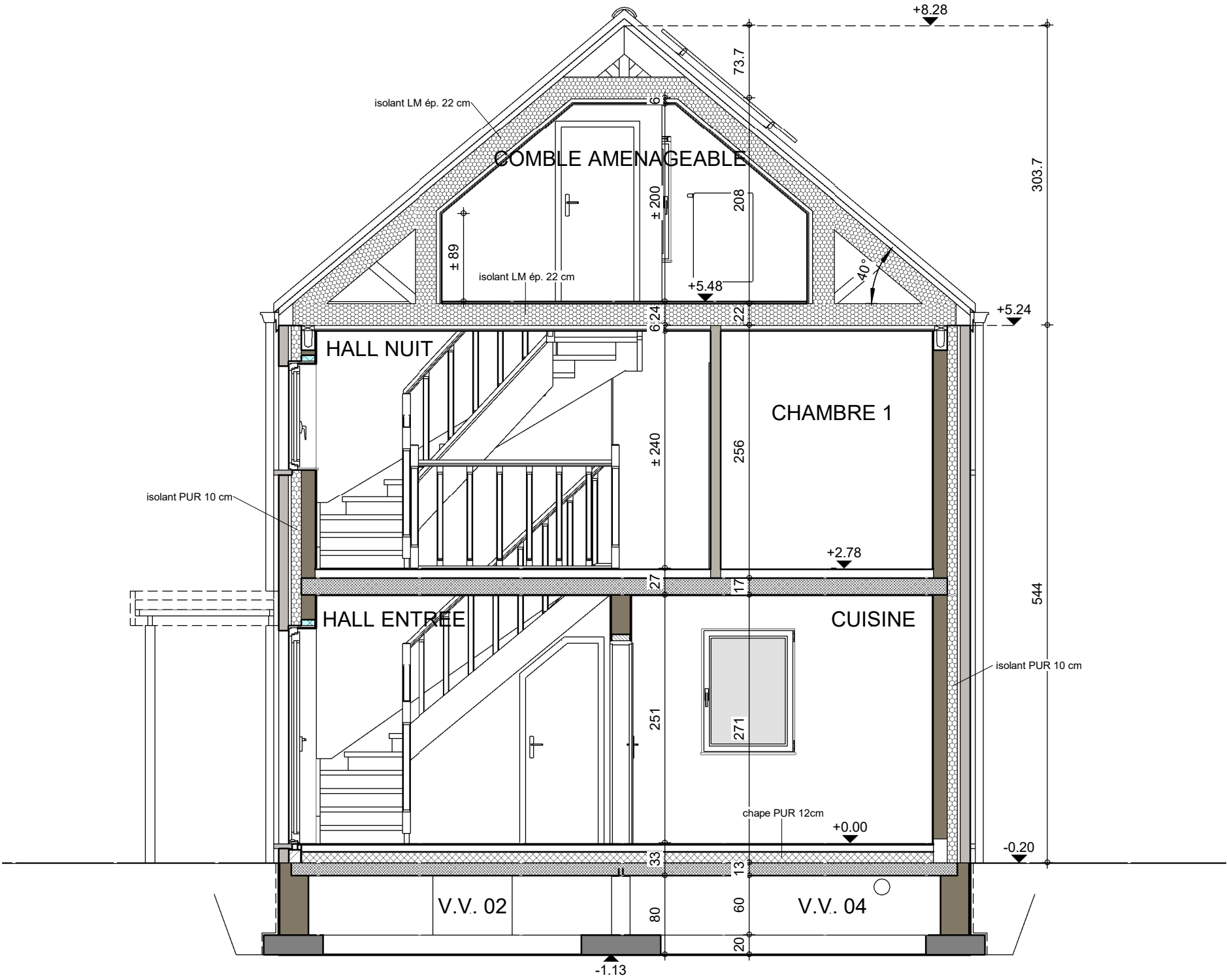
COUPE AA
