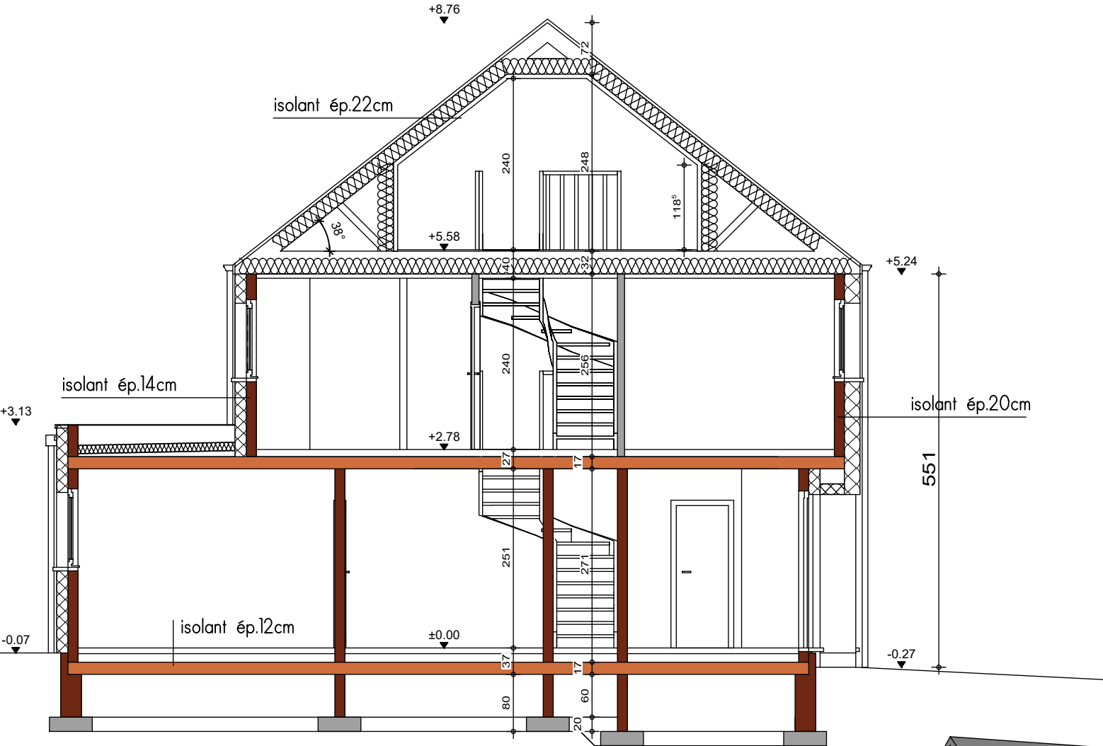
COUPE AA
