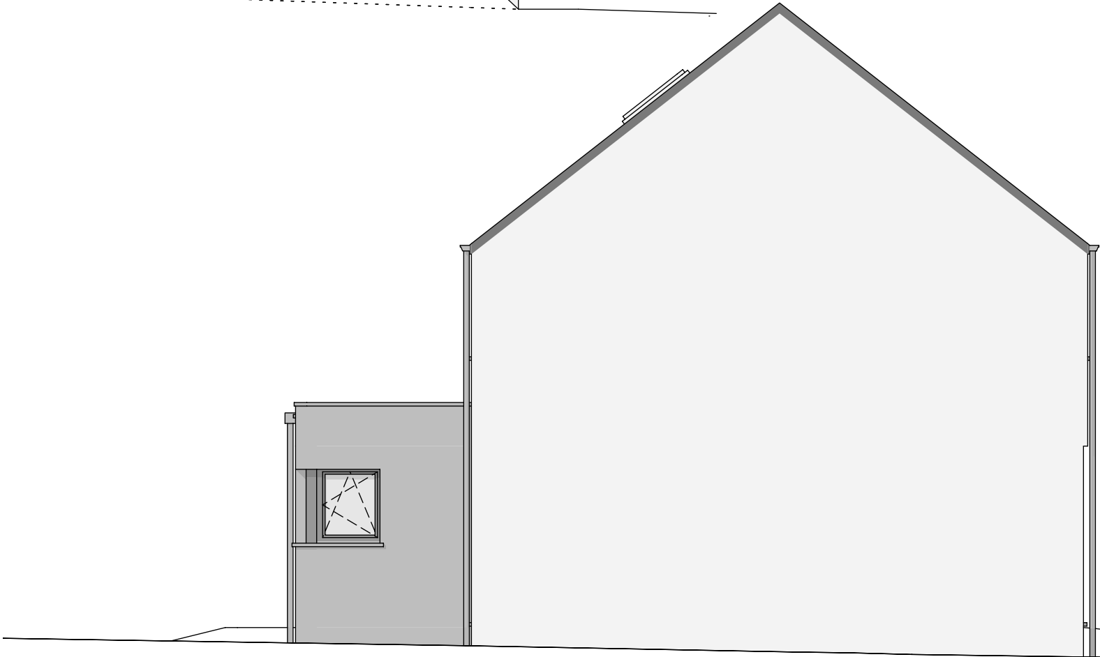
PIGNON GAUCHE
