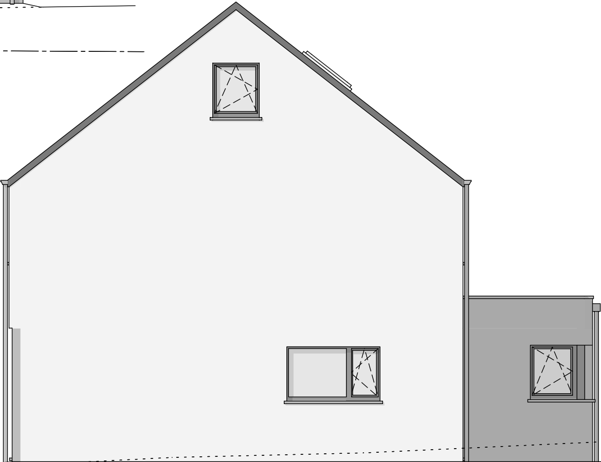
PIGNON DROIT
