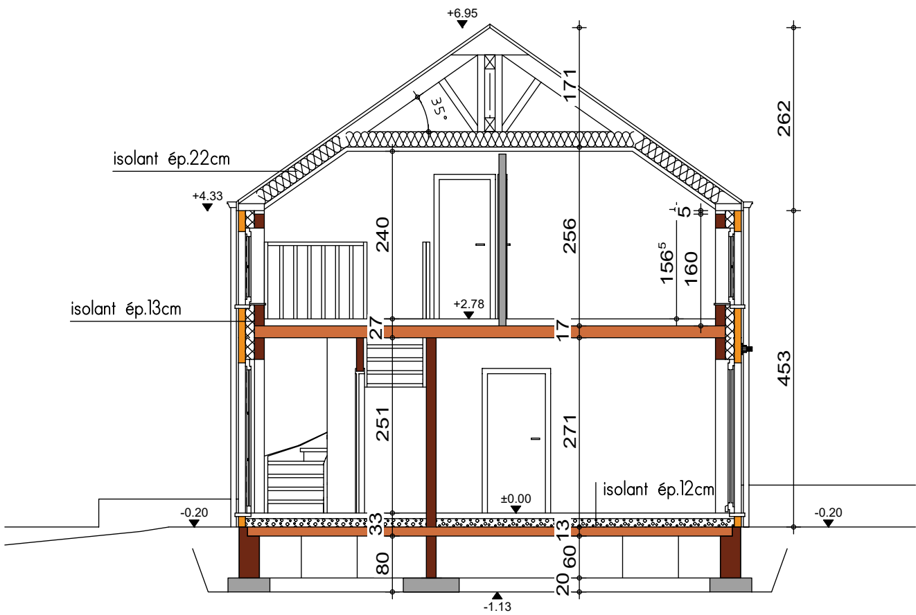
COUPE AA
