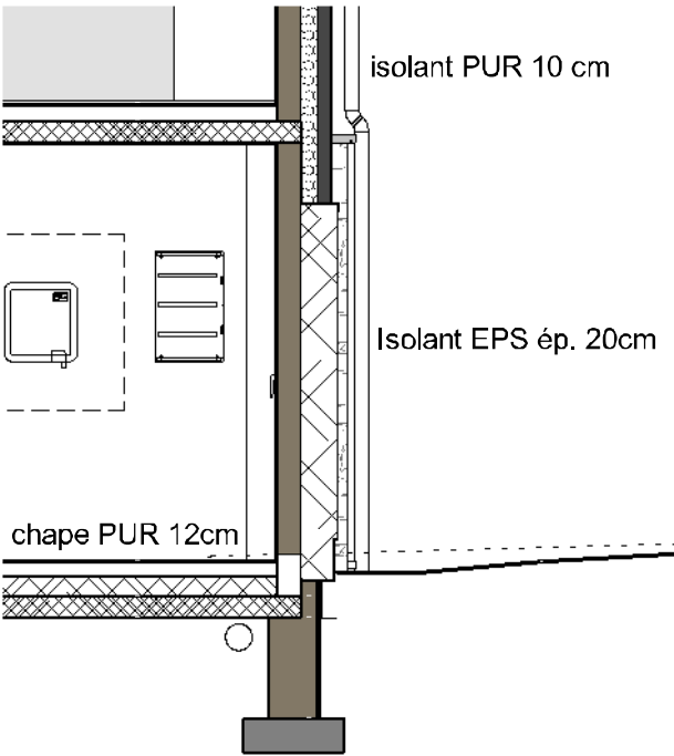
COUPE BB
