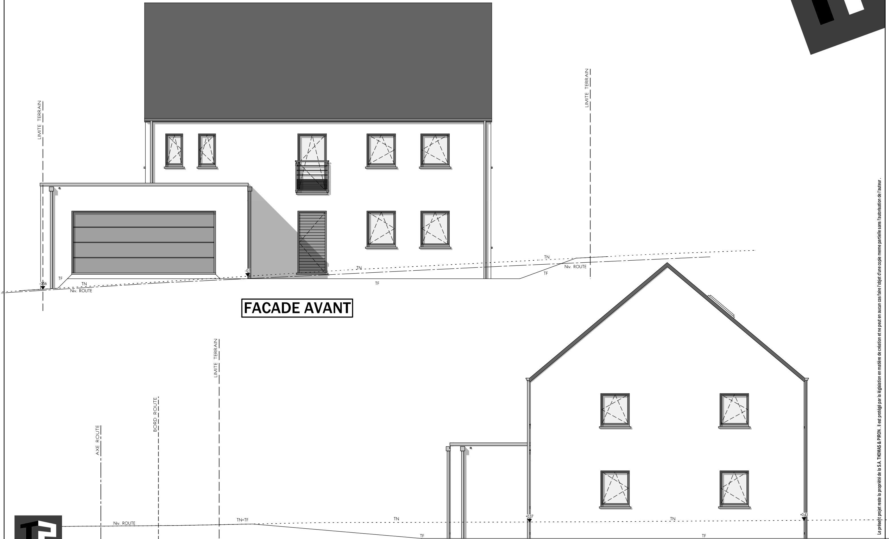
PIGNON DROIT
