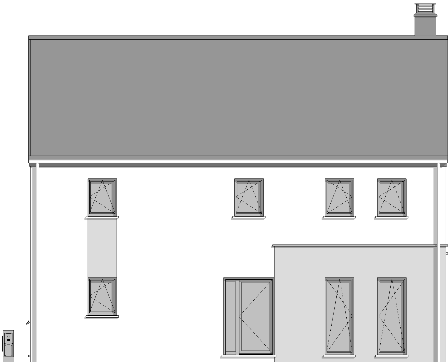
FACADE AVANT
