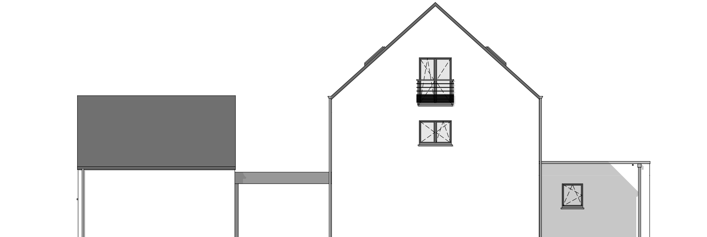
PIGNON DROIT
