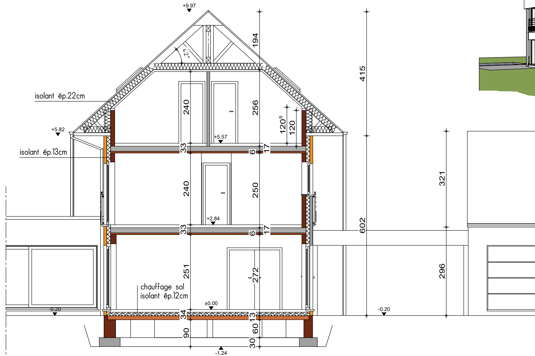
COUPE AA
