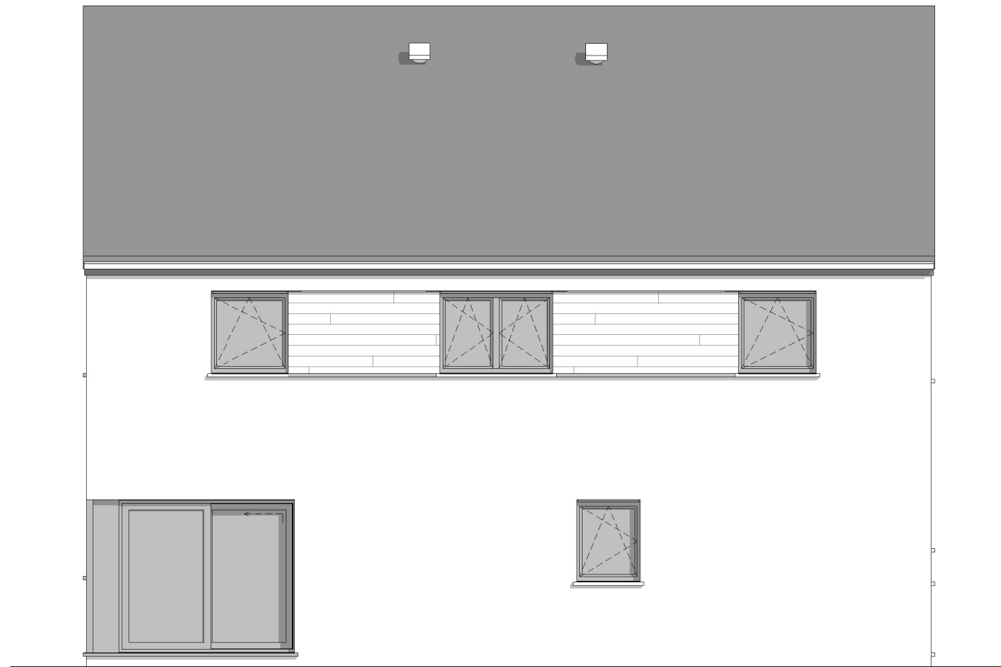
FACADE LATERALE GAUCHE
