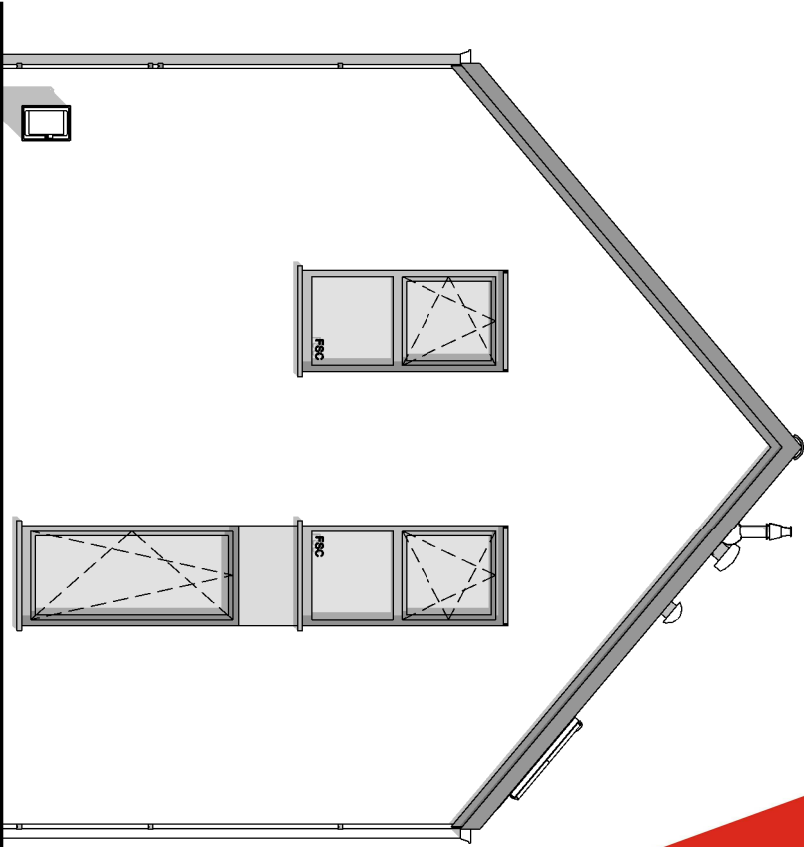
PIGNON DROIT
