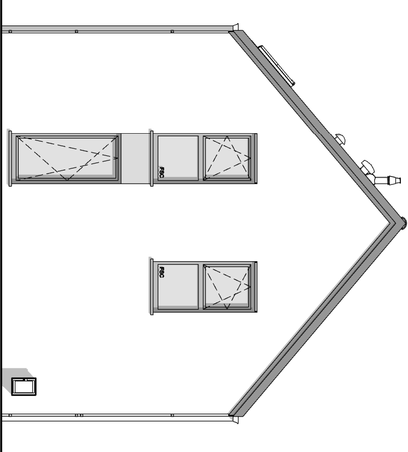
PIGNON GAUCHE
