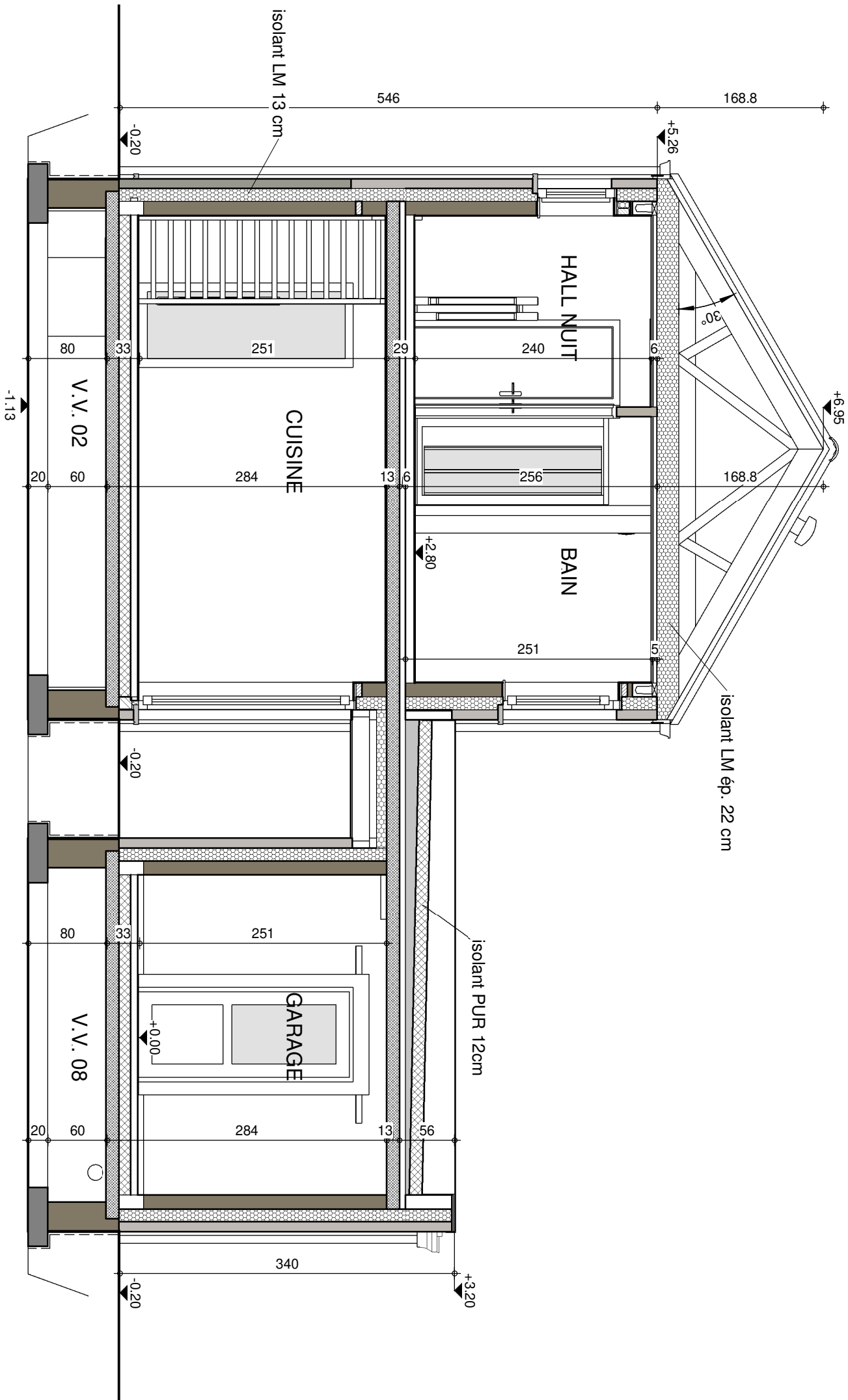
COUPE AA
