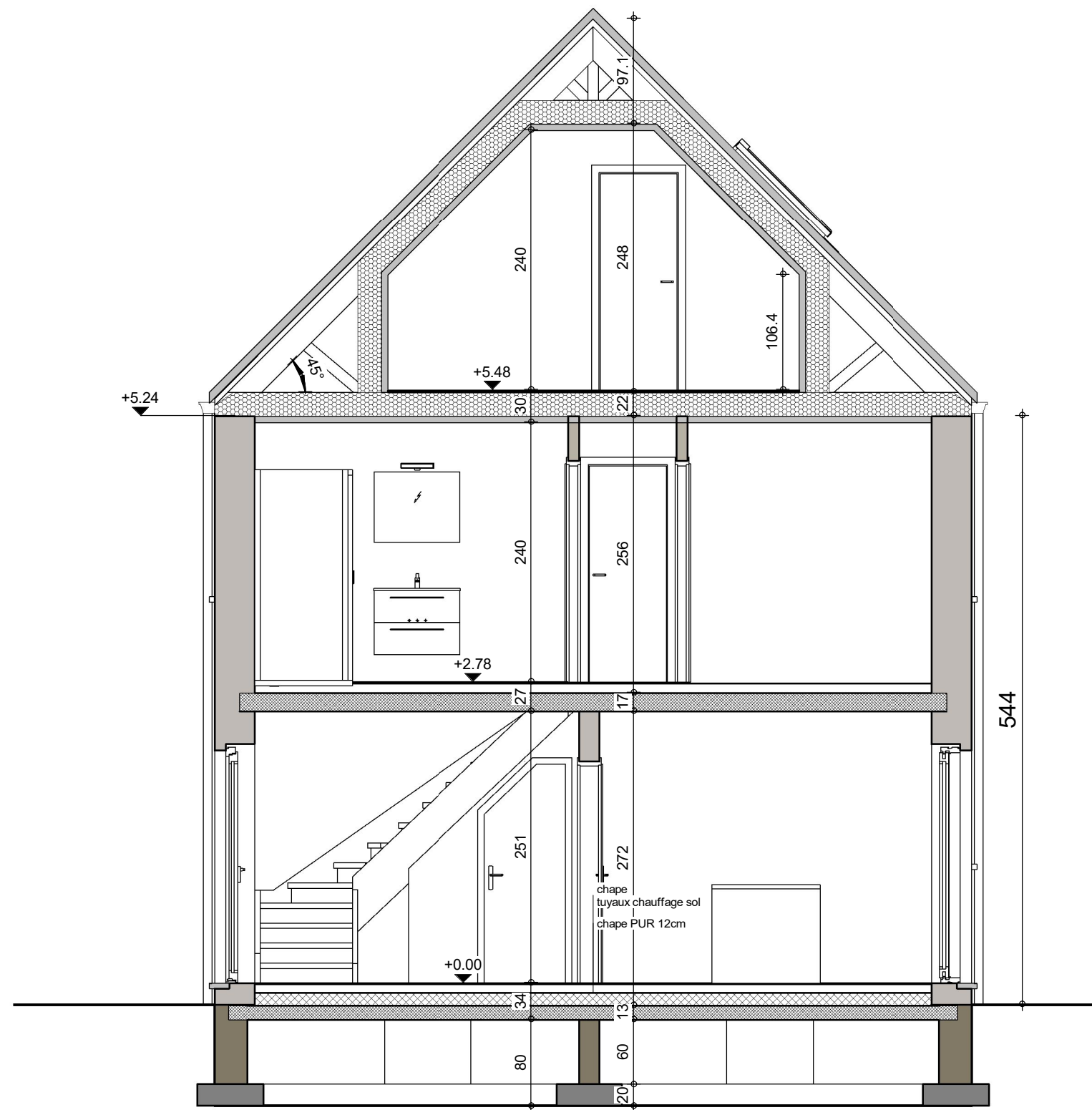
COUPE AA
