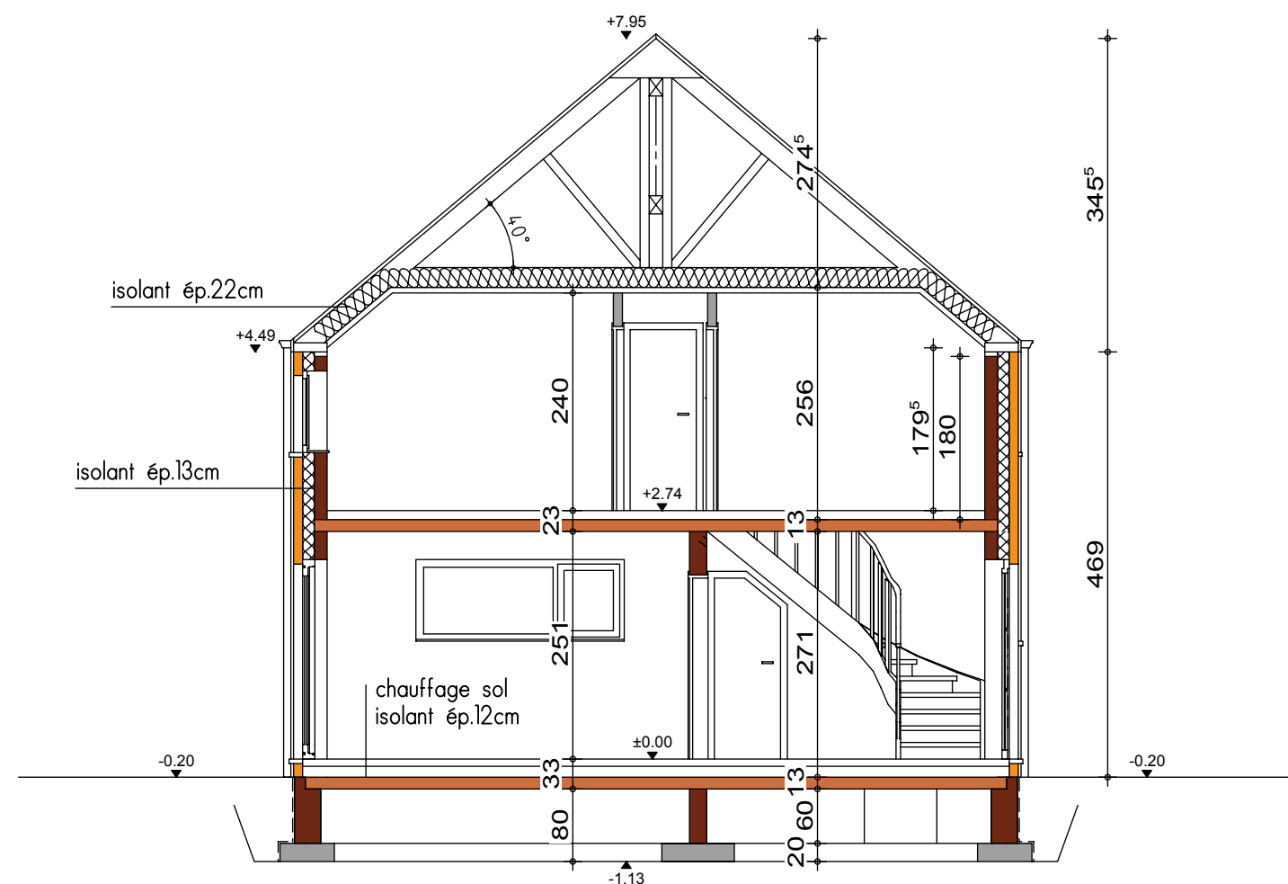
COUPE AA
