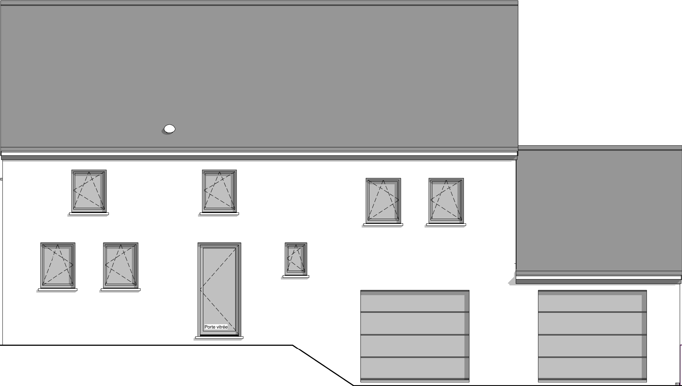
FACADE AVANT
