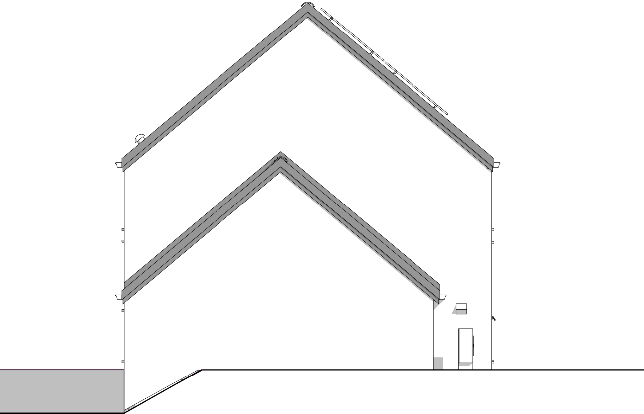
PIGNON DROIT
