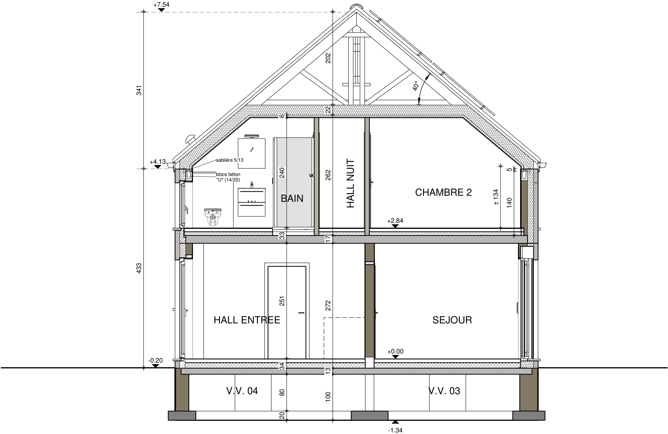
COUPE AA
