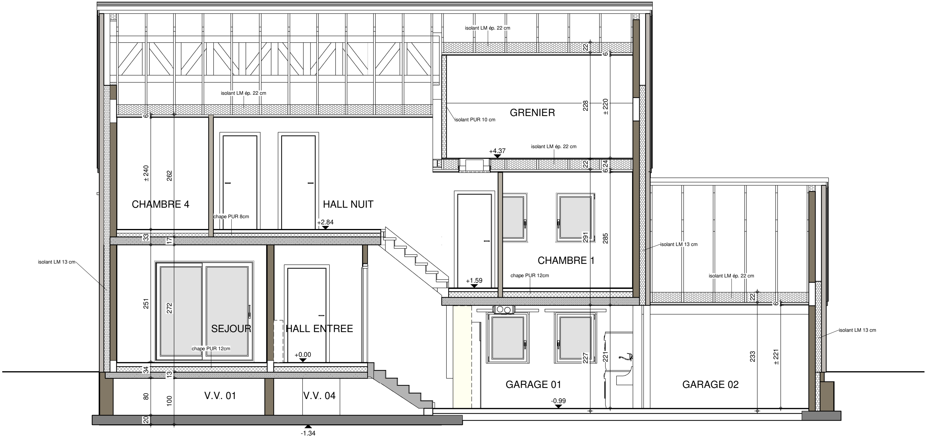
COUPE BB
