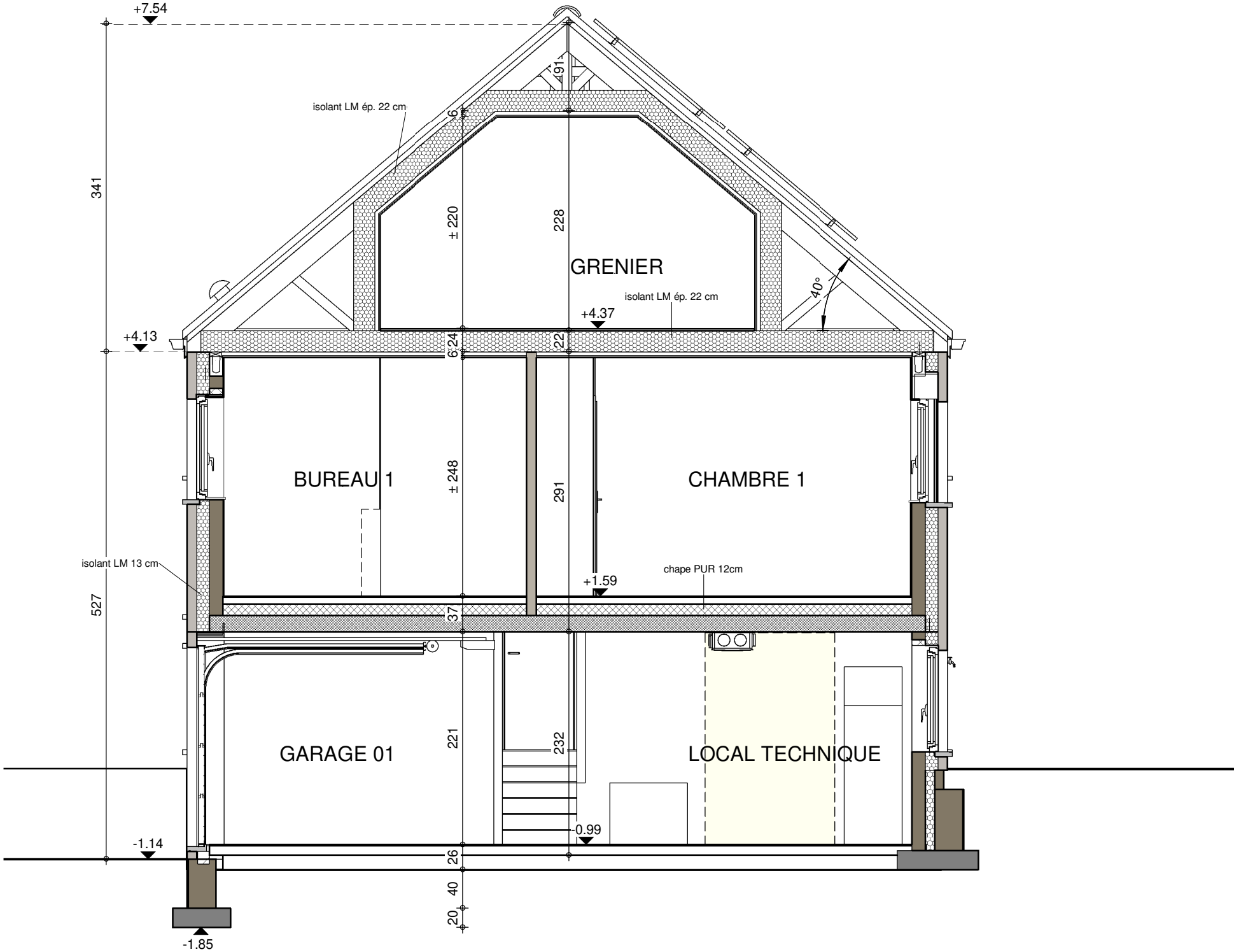
COUPE CC
