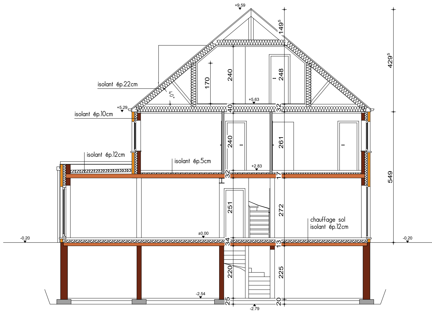
COUPE AA
