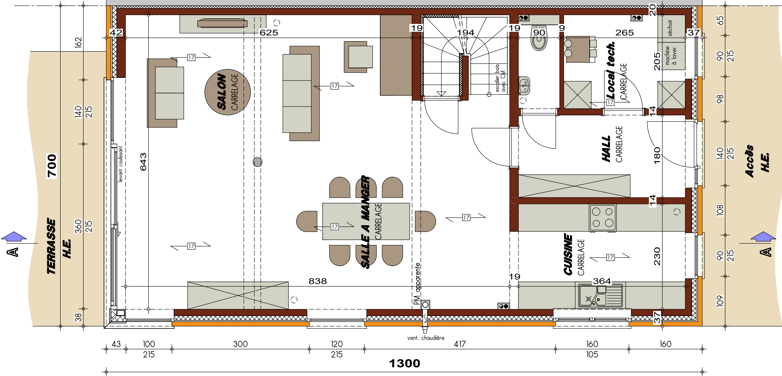
PLAN REZ-DE-CHAUSSEE
