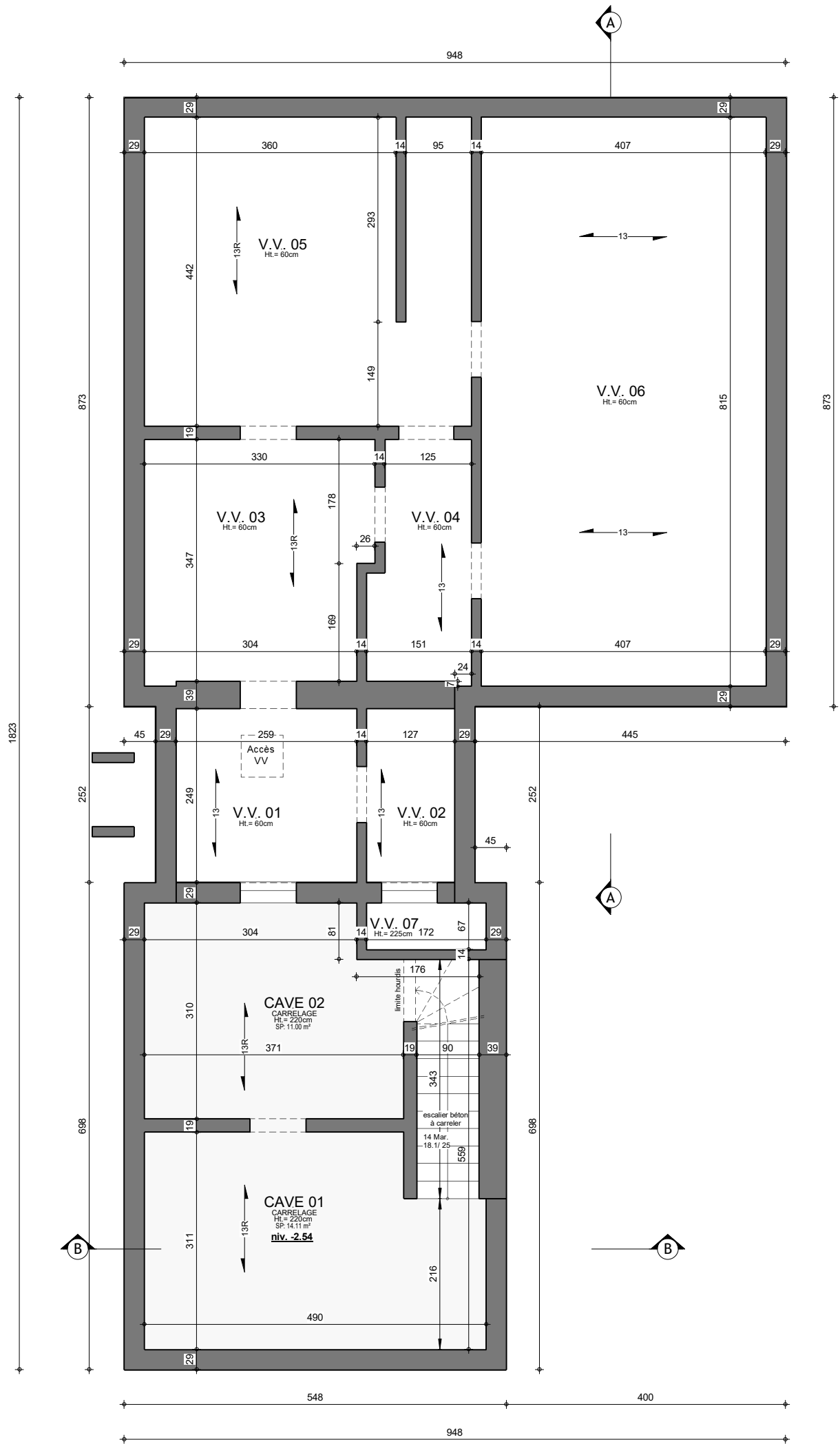
SOUS-SOL : Egouttage
