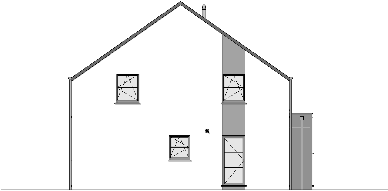
PIGNON GAUCHE
