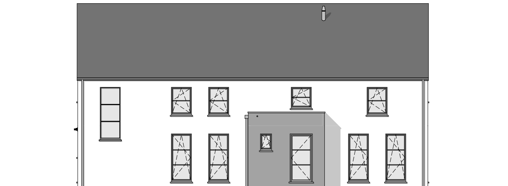
FACADE AVANT
