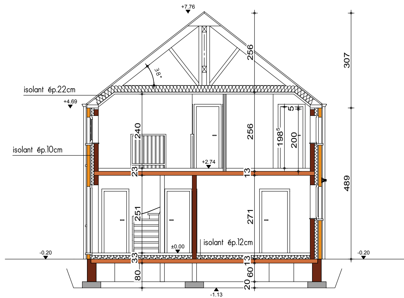
COUPE AA
