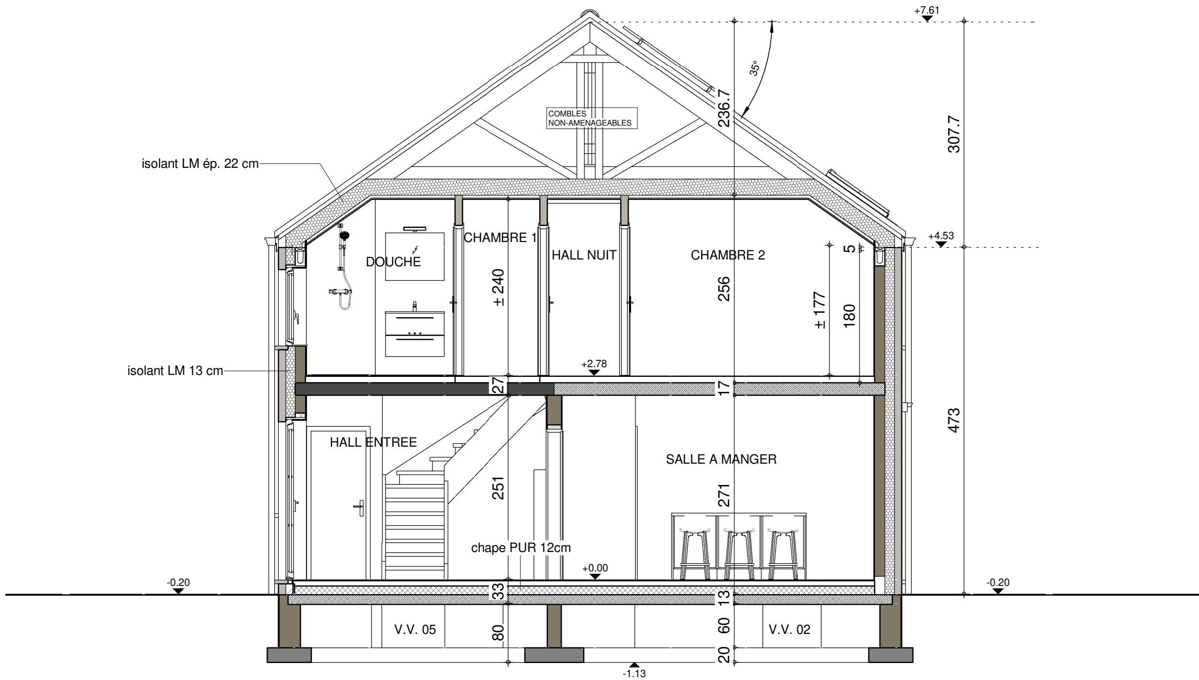
COUPE AA
